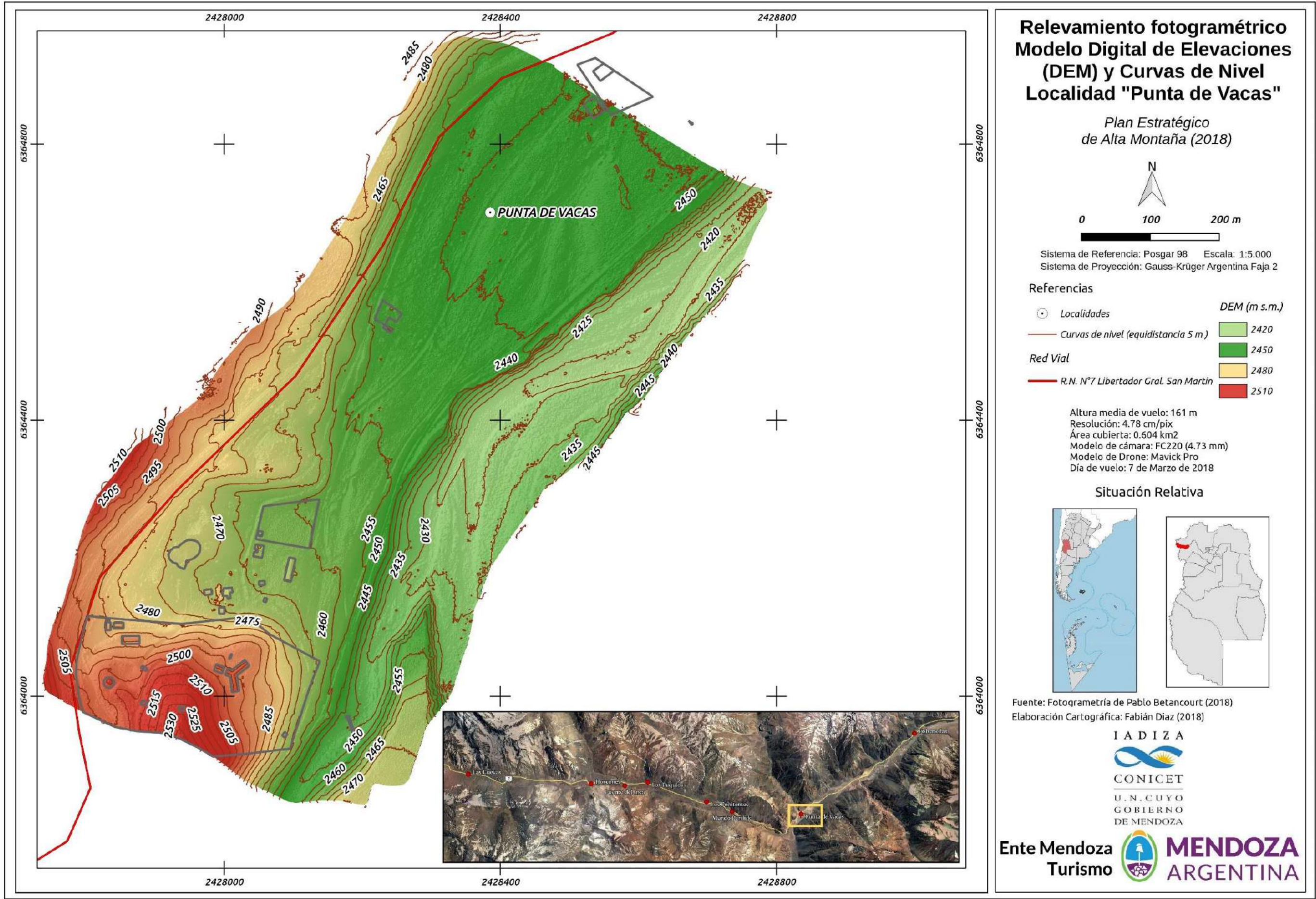
Figura 99. Relevamiento fotogramétrico. Modelo Digital de Elevaciones (MDE) y Curvas de Nivel. Localidad de Punta de Vacas – Sector oeste-.
