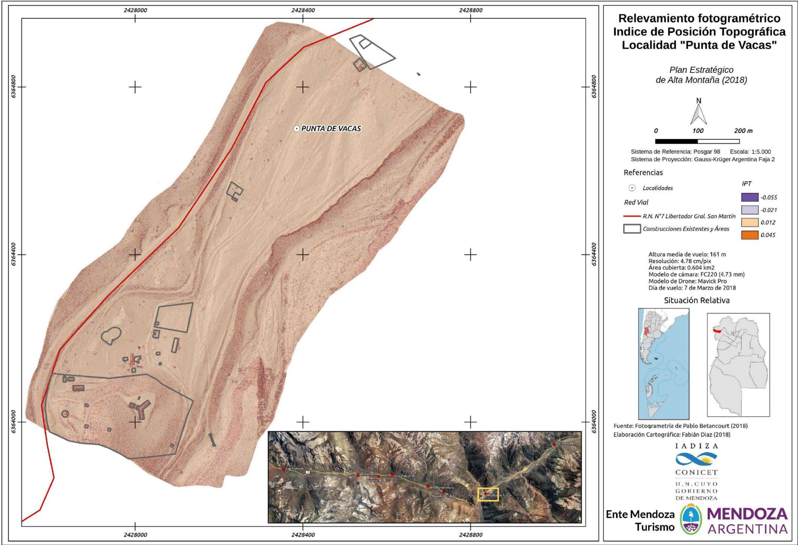
Figura 102. Relevamiento fotogramétrico. Índice de Posición Topográfica. Localidad de Punta de Vacas – Sector oeste-.
