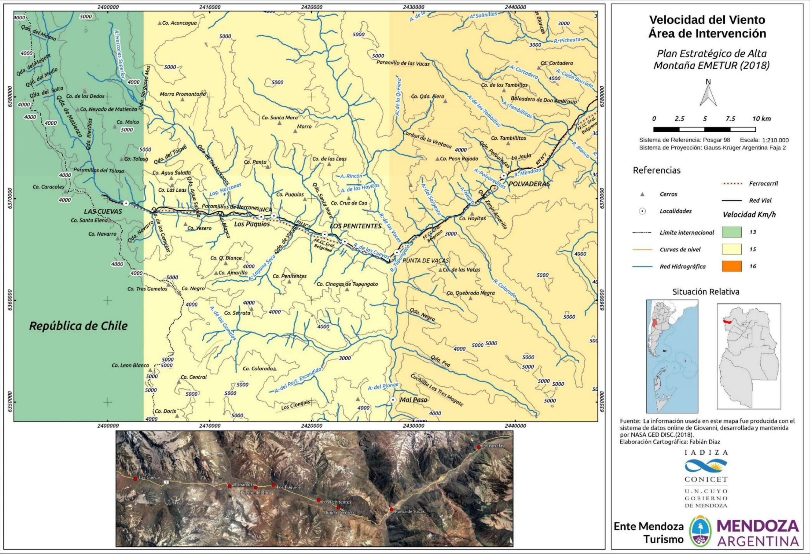
Figura 41. Velocidad del viento. Al del PEAM. Fuente: NASA GED DISC (2018)
