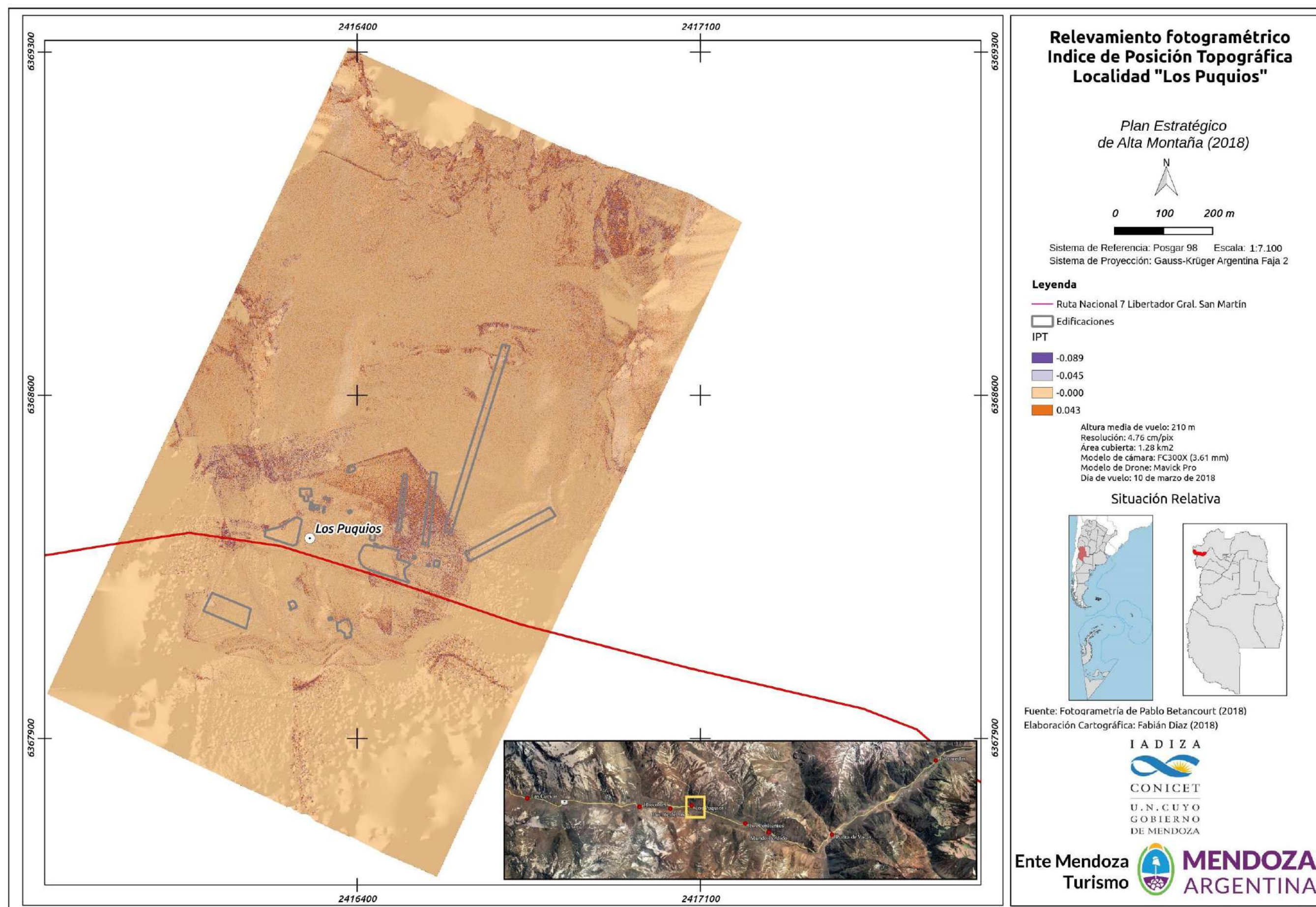
Figura 147. Relevamiento fotogramétrico. Índice de Posición Topográfica. Paraje "Los Puquios".
