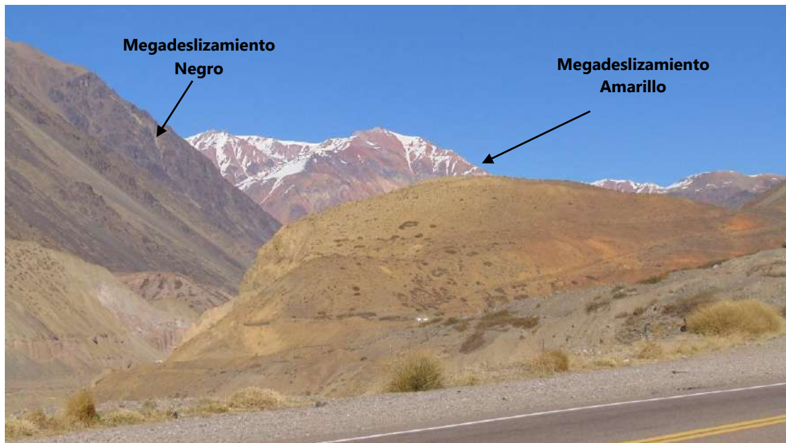
Figura 26. Deslizamientos pleistocénicos Amarillo y Negro. Valle del río Horcones.
