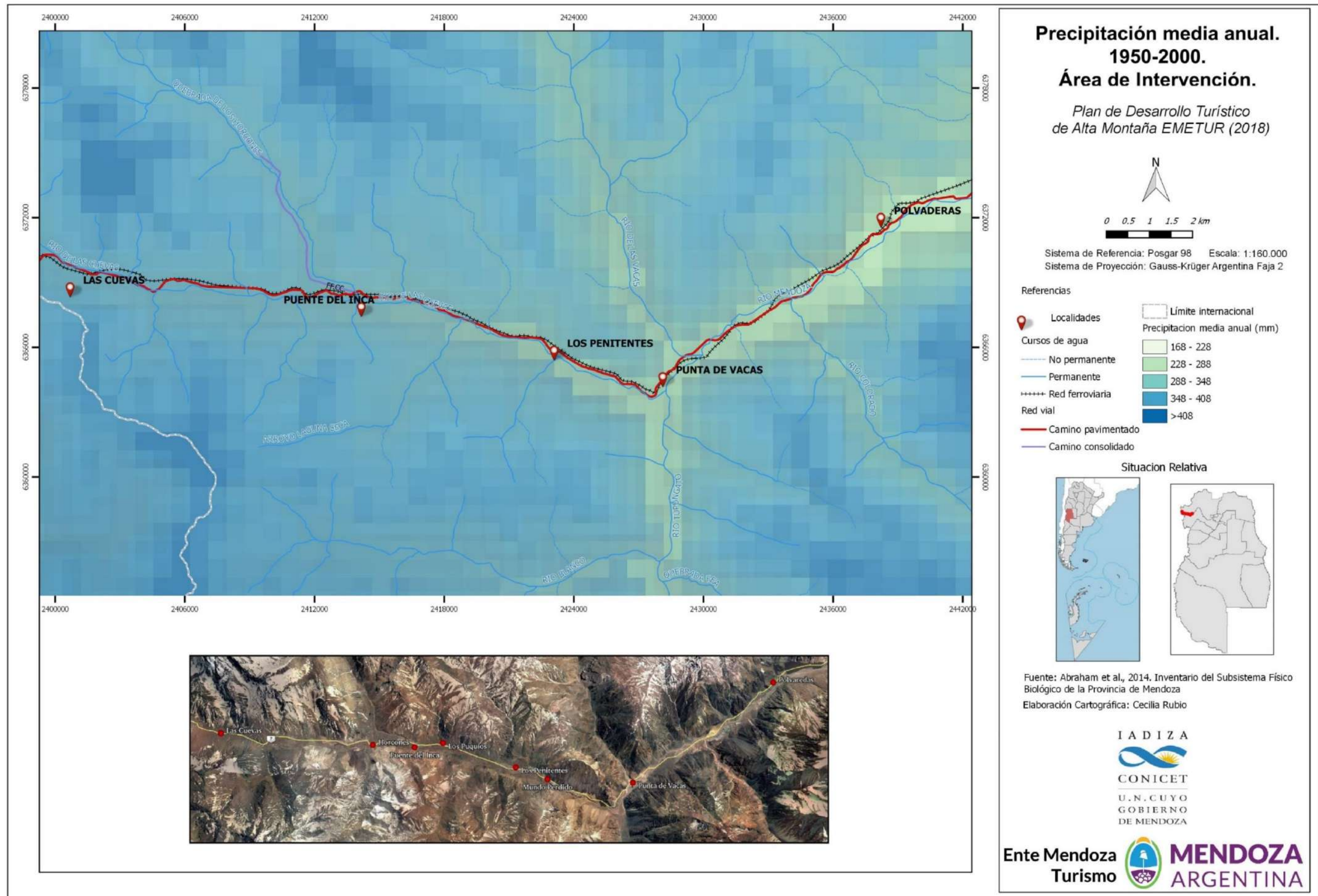
Figura 39. Precipitación media anual del AI del PEAM. Fuente: Abraham et al. (2014)
