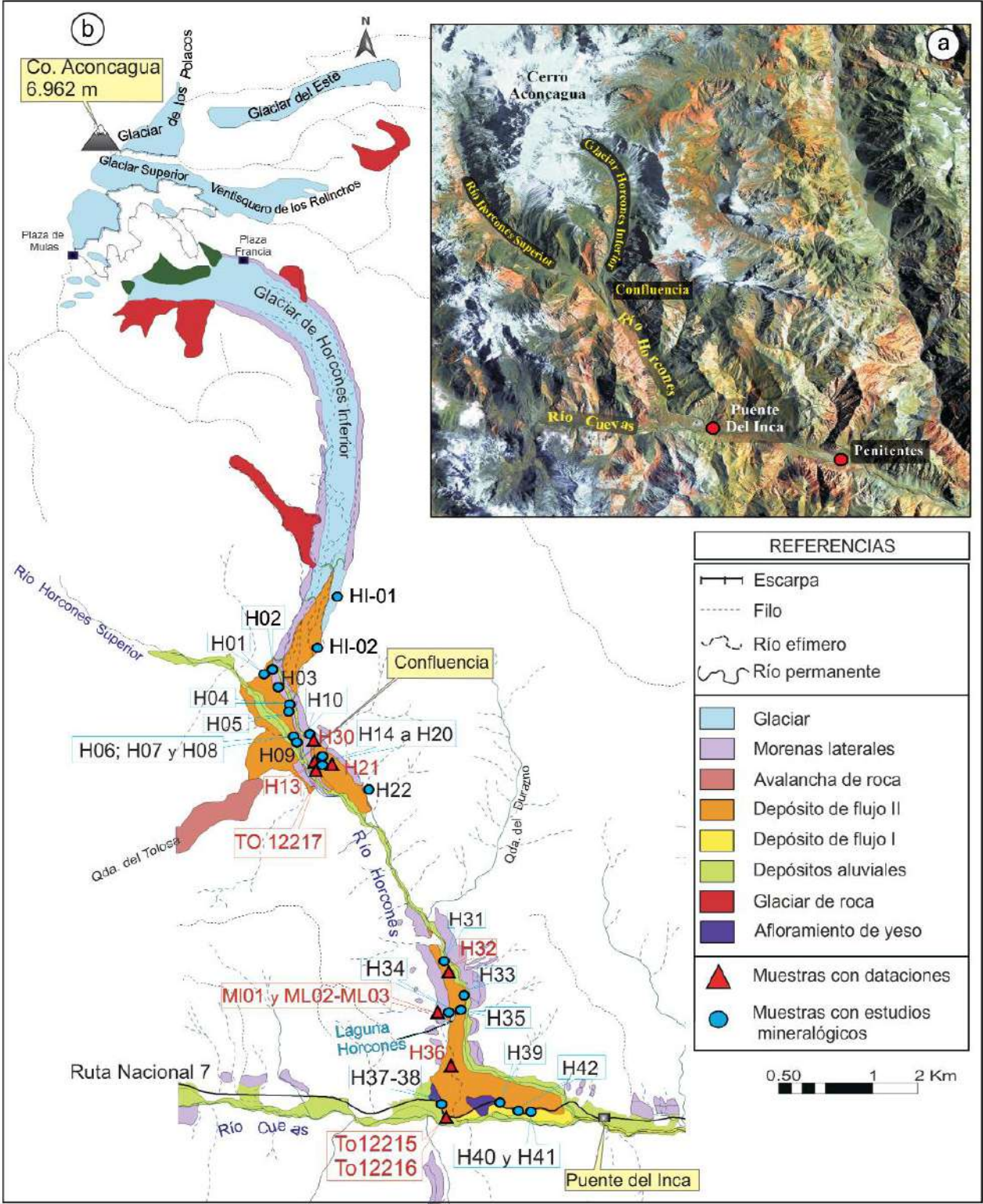
Figura 22. Mapa de unidades cuaternarias en el Parque Provincial Aconcagua. Localización del glaciar de Horcones Superior e Inferior, glaciar de los Polacos, glaciar del Este y el ventisquero de los Relinchos.
