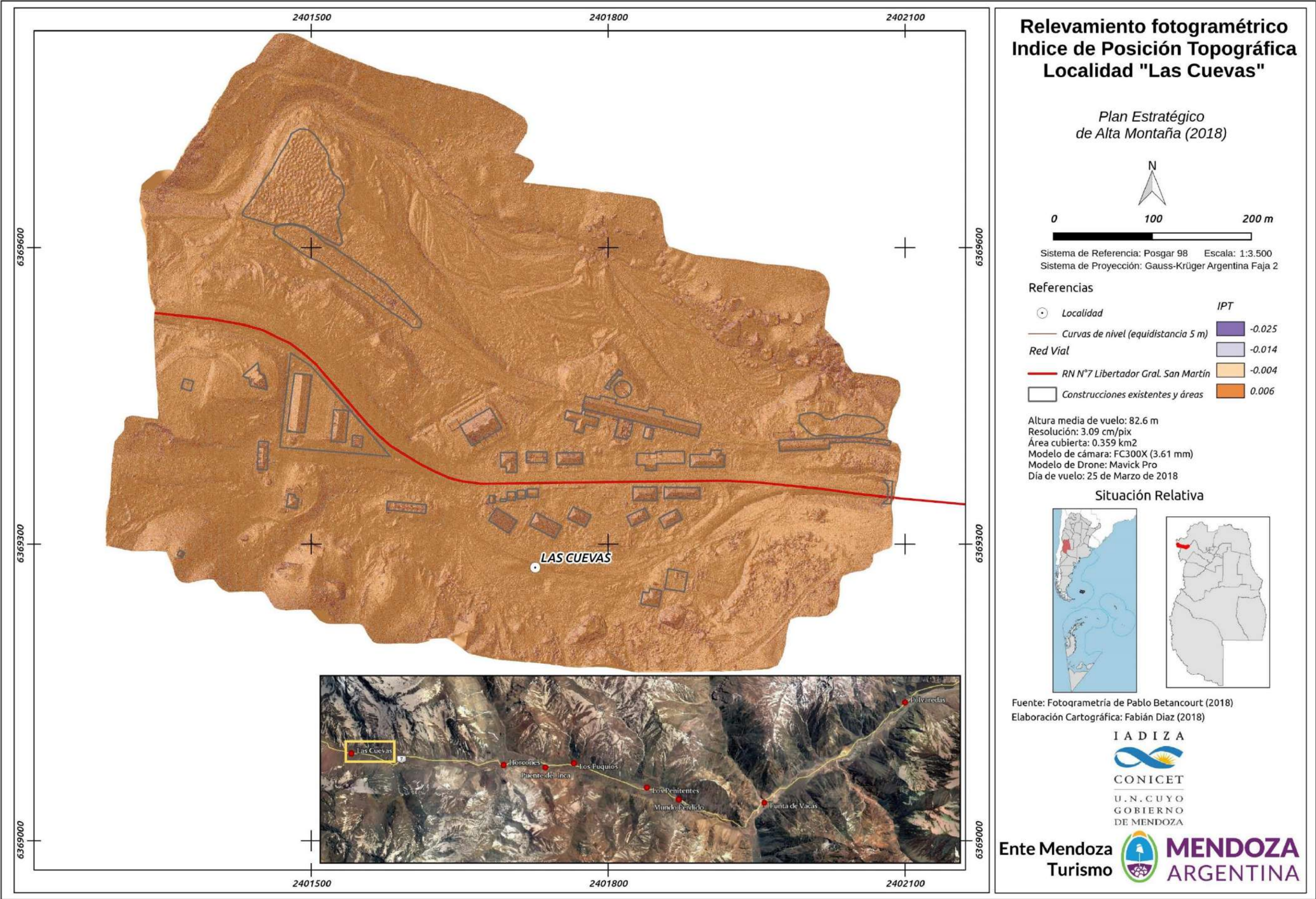
Figura 178. Relevamiento fotogramétrico. Índice de Posición Topográfica. Localidad "Las Cuevas".
