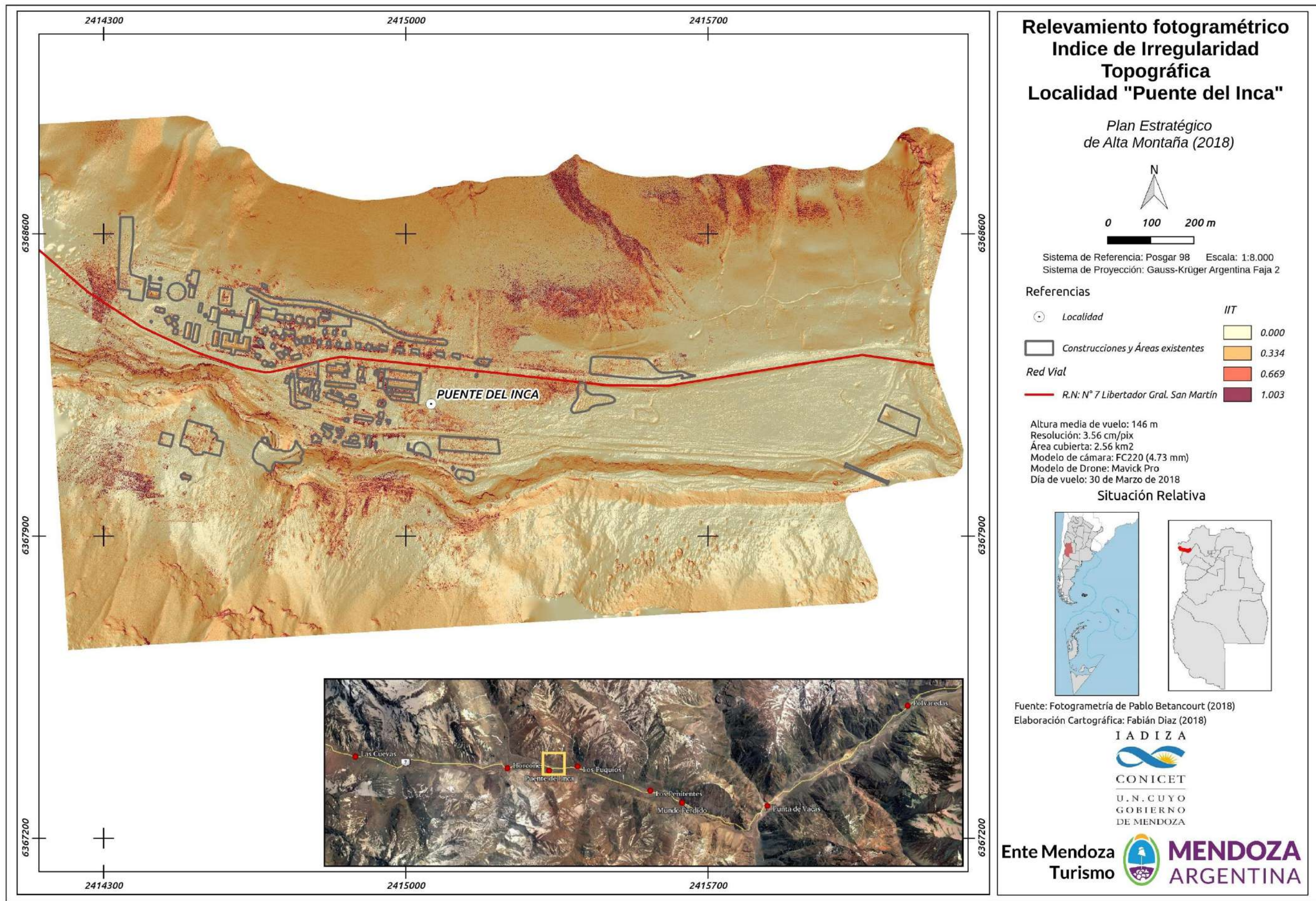
Figura 164. Relevamiento fotogramétrico. Índice de Irregularidad Topográfica. Localidad "Puente del Inca".
