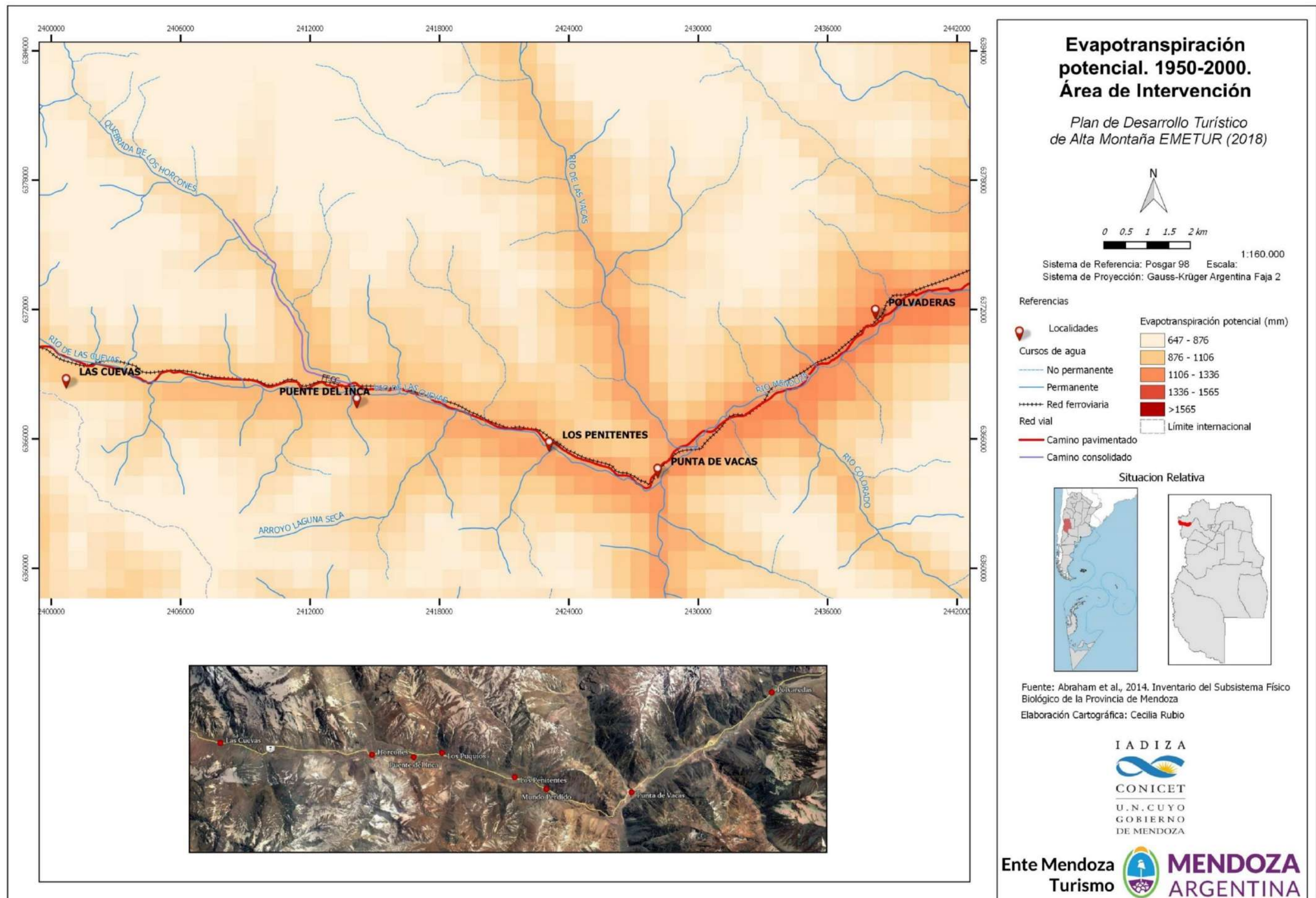
Figura 40. Evapotranspiración potencial del AI del PEAM. Fuente: Abraham et al. (2014)
