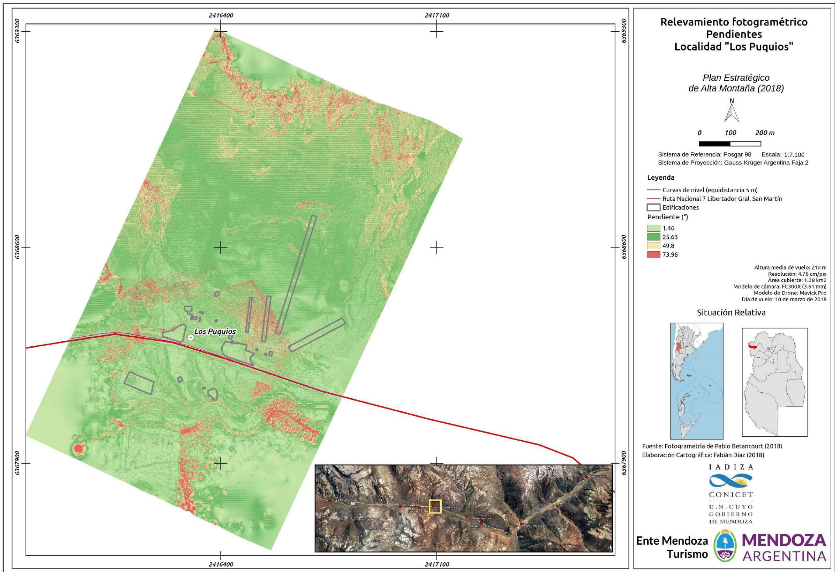
Figura 145. Relevamiento fotogramétrico. Pendientes. Paraje "Los Puquios".
