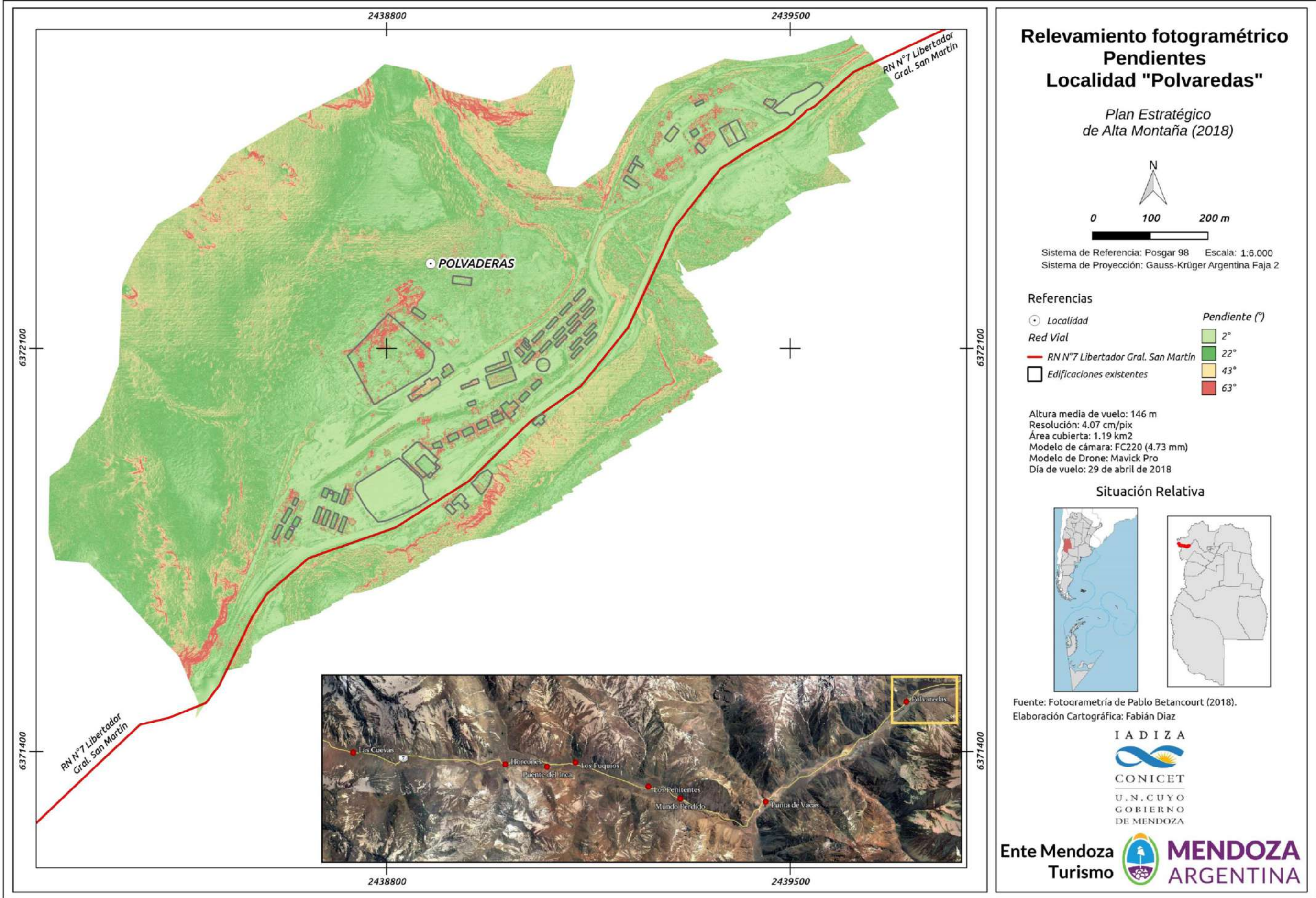
Figura 90. Relevamiento fotogramétrico. Pendientes. Localidad "Polvaredas".
