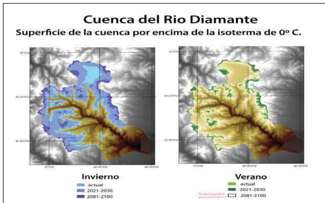
Figura 42. Cuenca del Río Diamante. Superficie de la cuenca por encima de la isoterma de 0°C.
