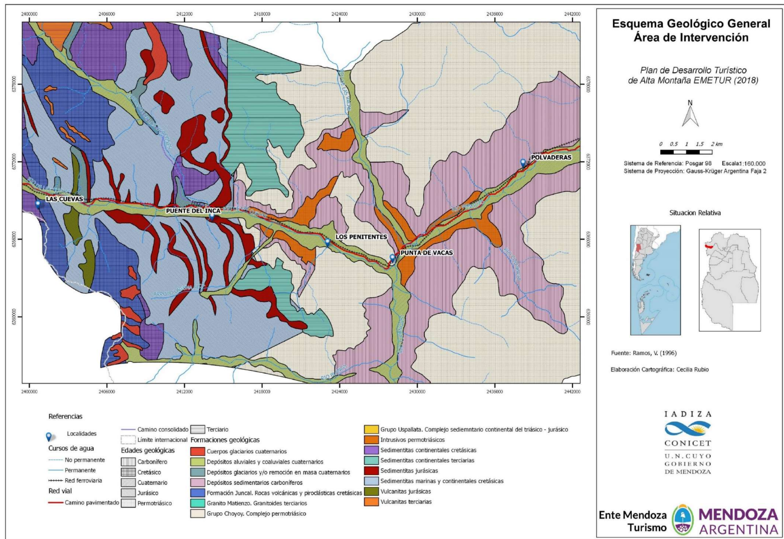
Figura 33. Esquema geológico general del AI del PEAM. Fuente: Ramos (1996)
