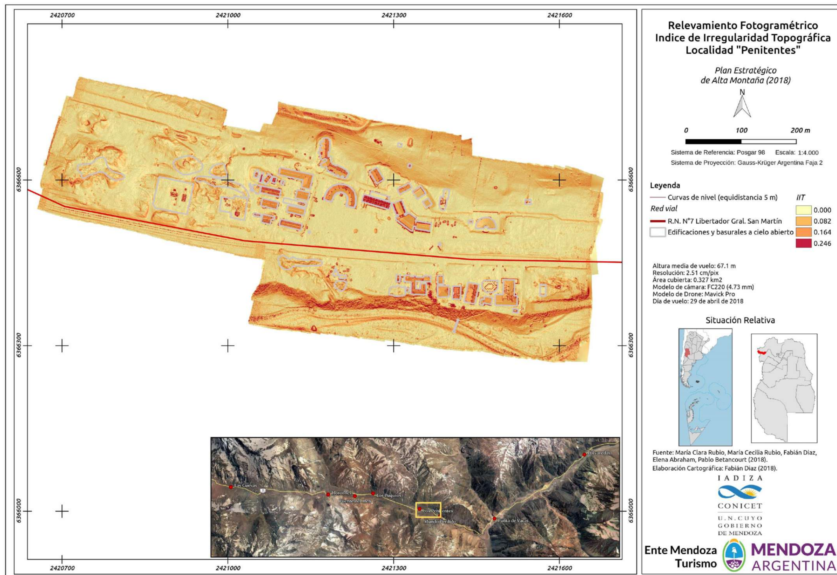
Figura 134. Relevamiento fotogramétrico. Índice de Irregularidad Topográfica. Localidad "Penitentes".
