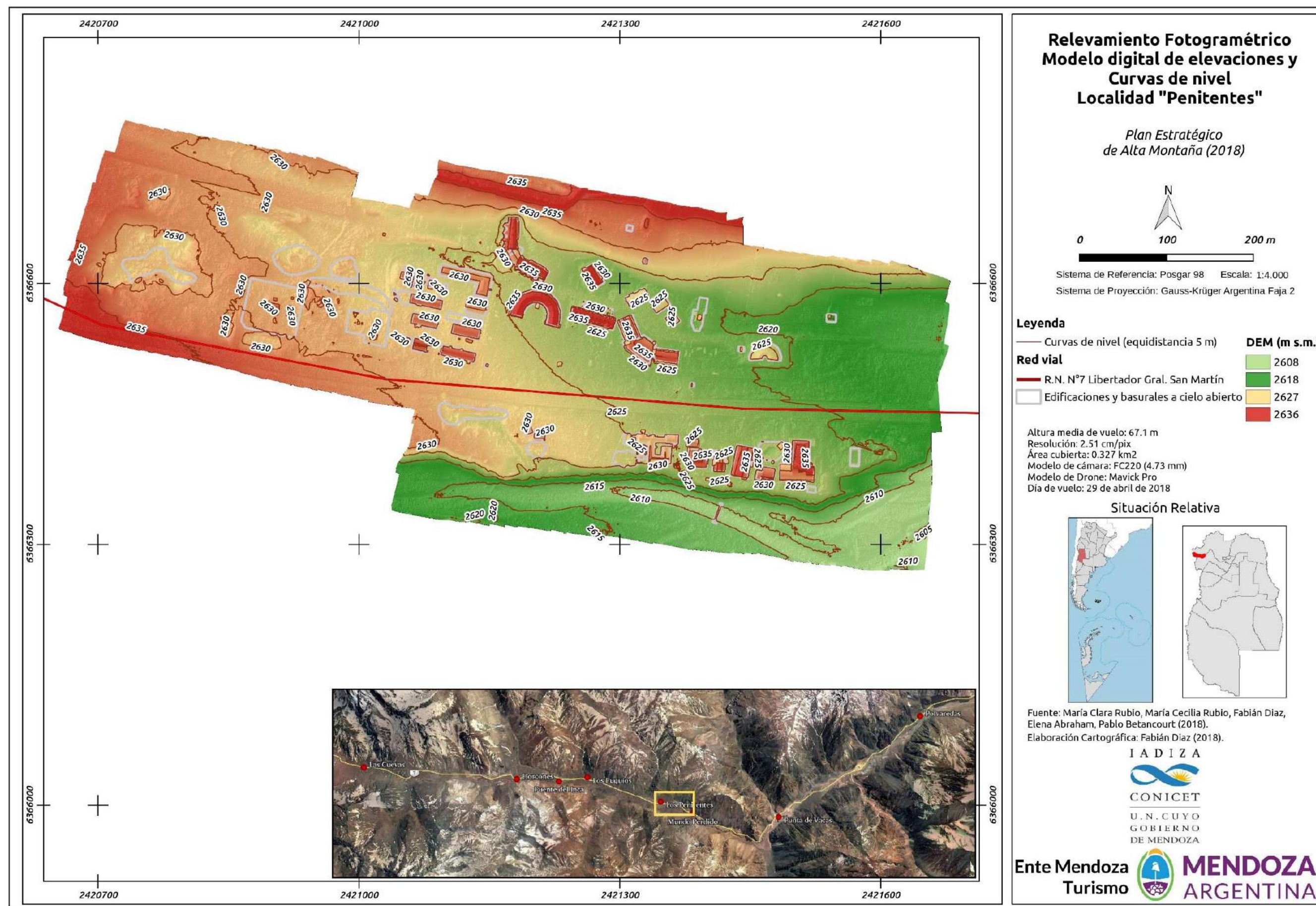
Figura 130. Relevamiento fotogramétrico. Modelo Digital de Elevaciones (MDE) y Curvas de nivel. Localidad "Penitentes".
