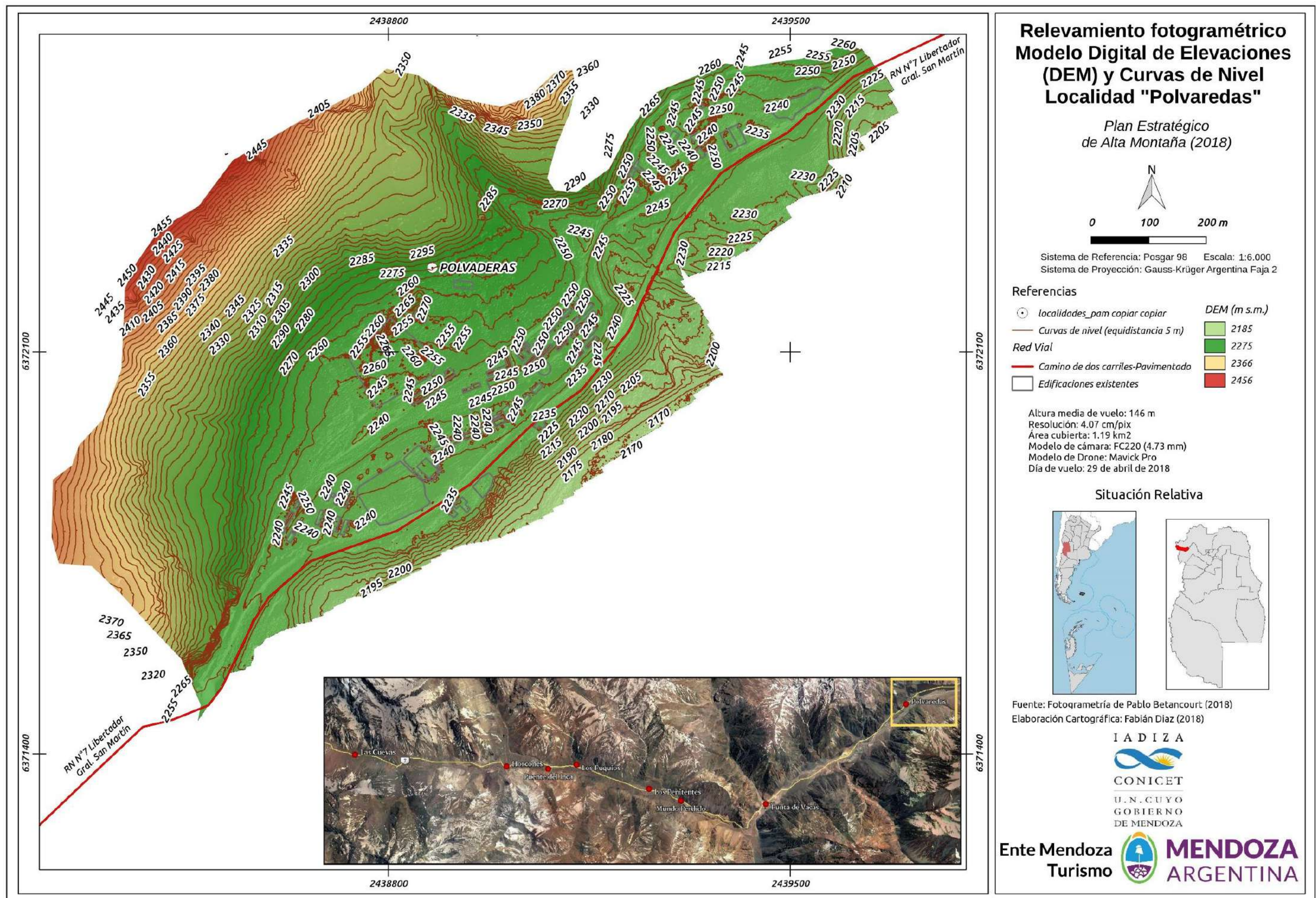
Figura 89. Relevamiento fotogramétrico. Modelo Digital de Elevaciones (DEM) y Curvas de Nivel. Localidad "Polvaredas".
