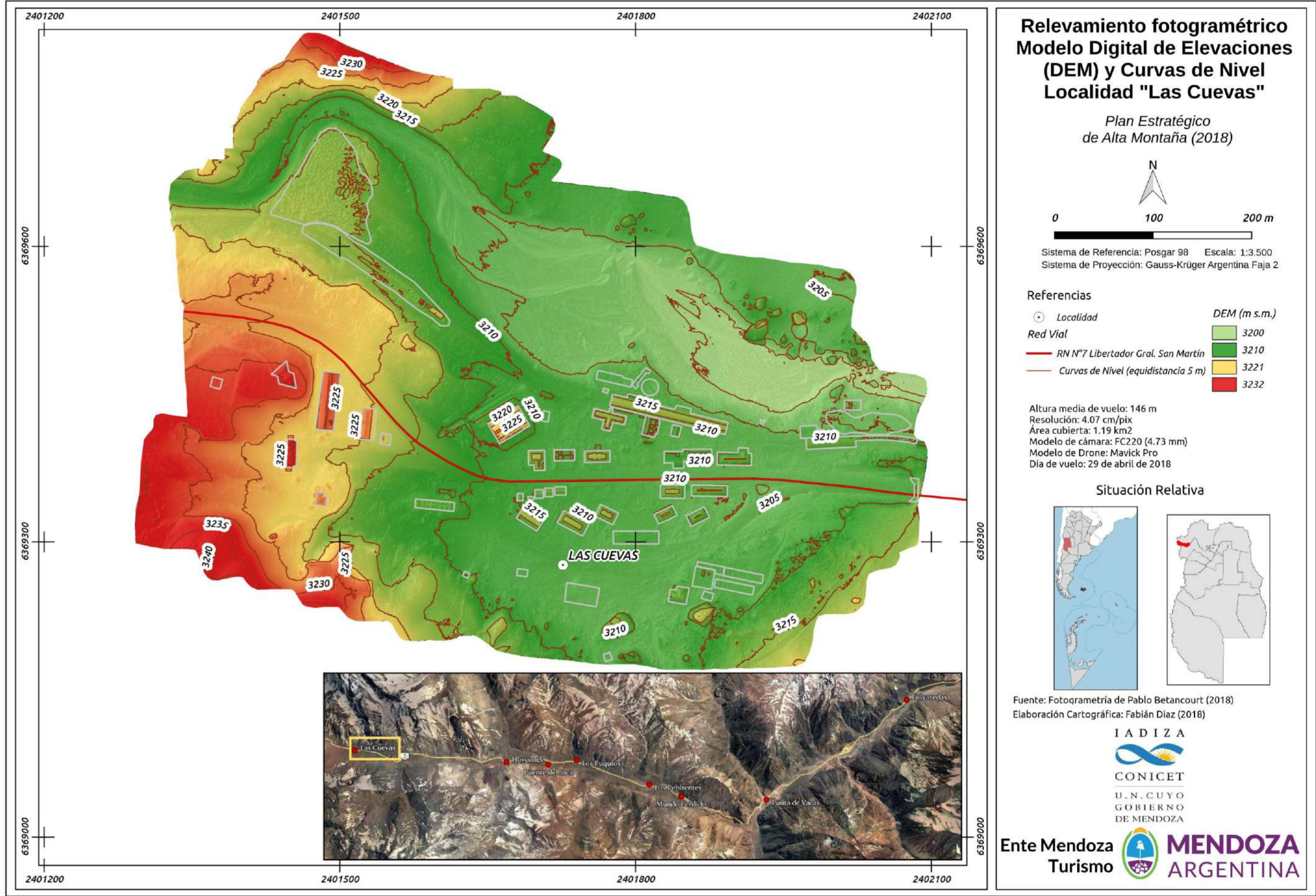
Figura 175. Relevamiento fotogramétrico. Modelo de Digital de Elevaciones (DEM) y Curvas de Nivel. Localidad "Las Cuevas".
