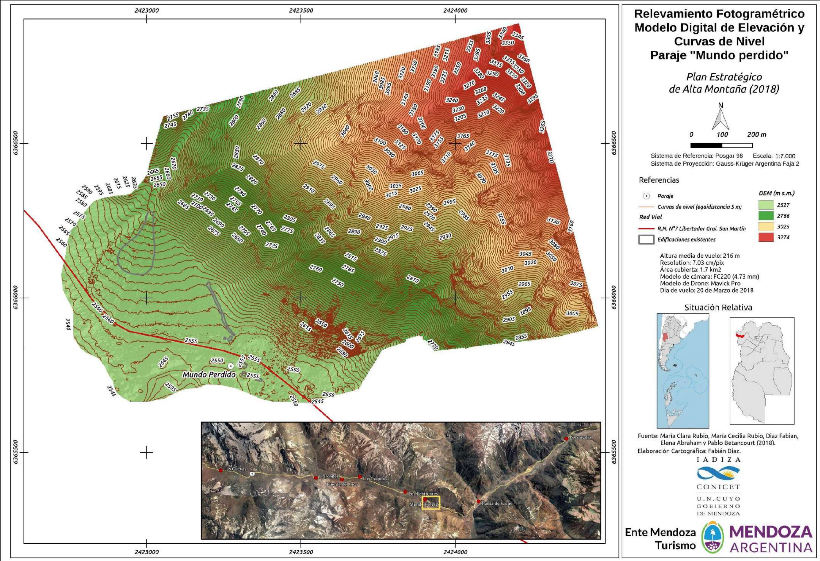
Figura 113. Relevamiento fotogramétrico. Modelo Digital de Elevación y Curvas de nivel. Paraje Km 151 "Mundo perdido" y "Pircas".
