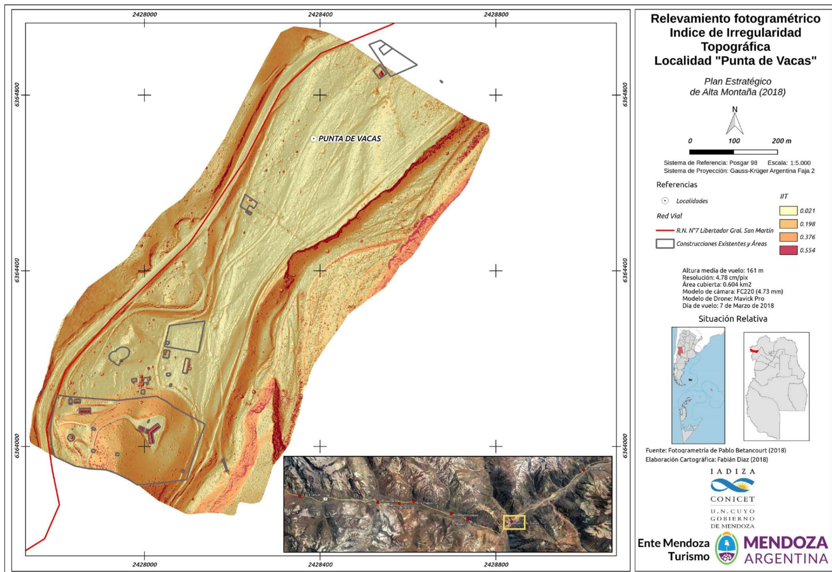
Figura 103. Relevamiento fotogramétrico. Índice de Irregularidad Topográfica. Localidad de Punta de Vacas – Sector oeste-.
