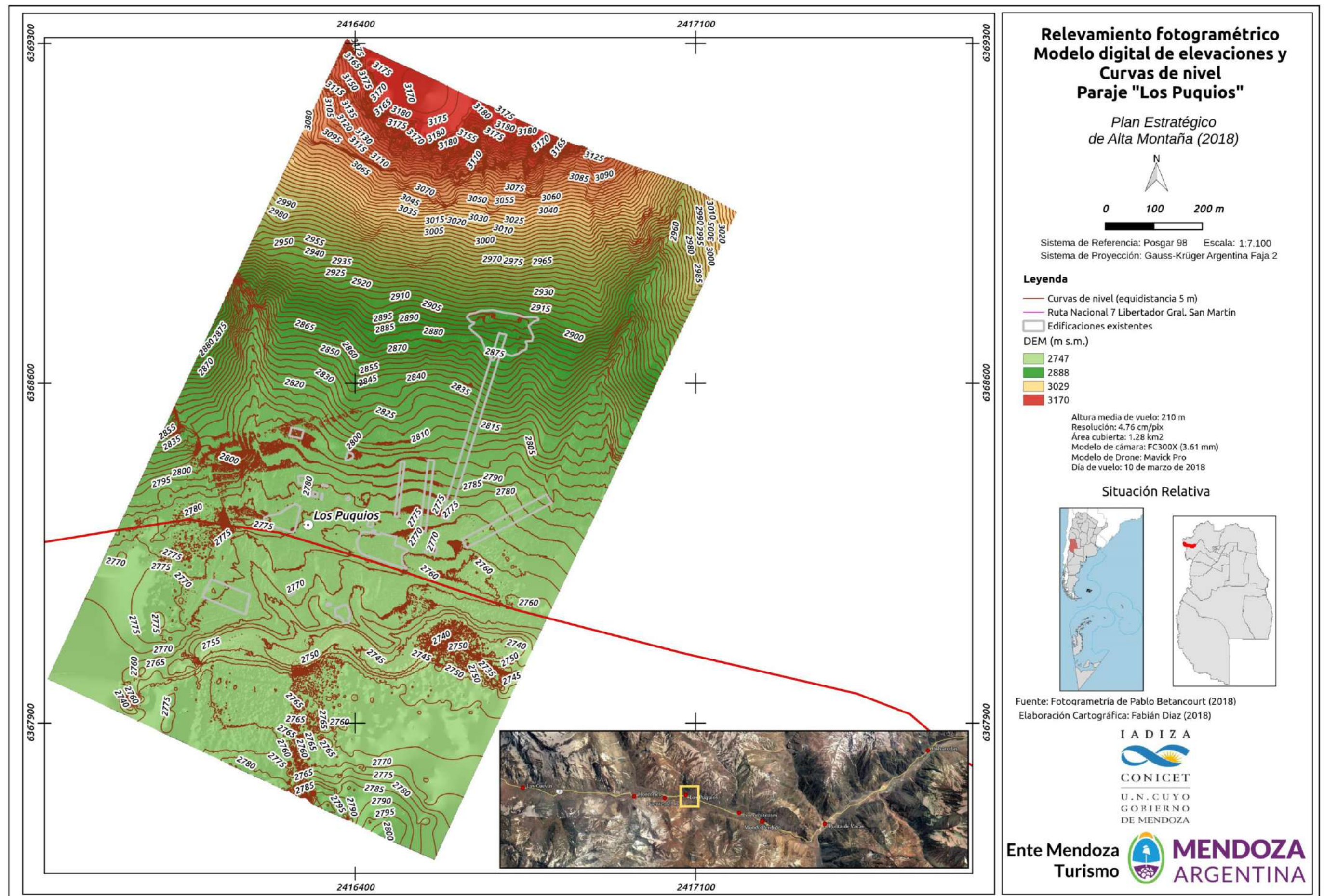
Figura 144. Relevamiento fotogramétrico. Modelo Digital de Elevaciones (MDE) y Curvas de Nivel. Paraje "Los Puquios".
