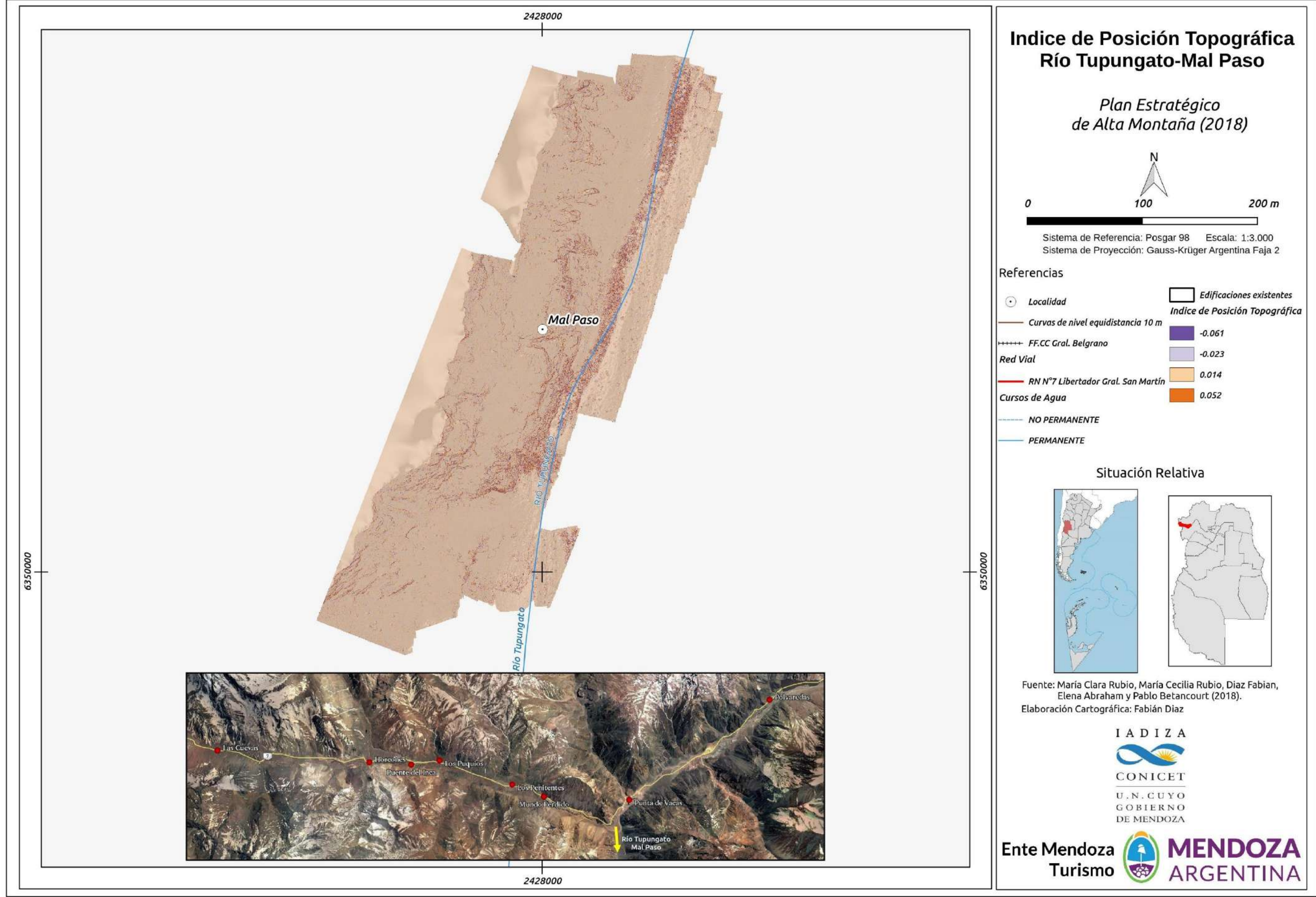
Figura 231. Relevamiento fotogramétrico. Índice de Posición Topográfica. Sitio natural de interés turístico “El mal paso” - Quebrada del río Tupungato.
