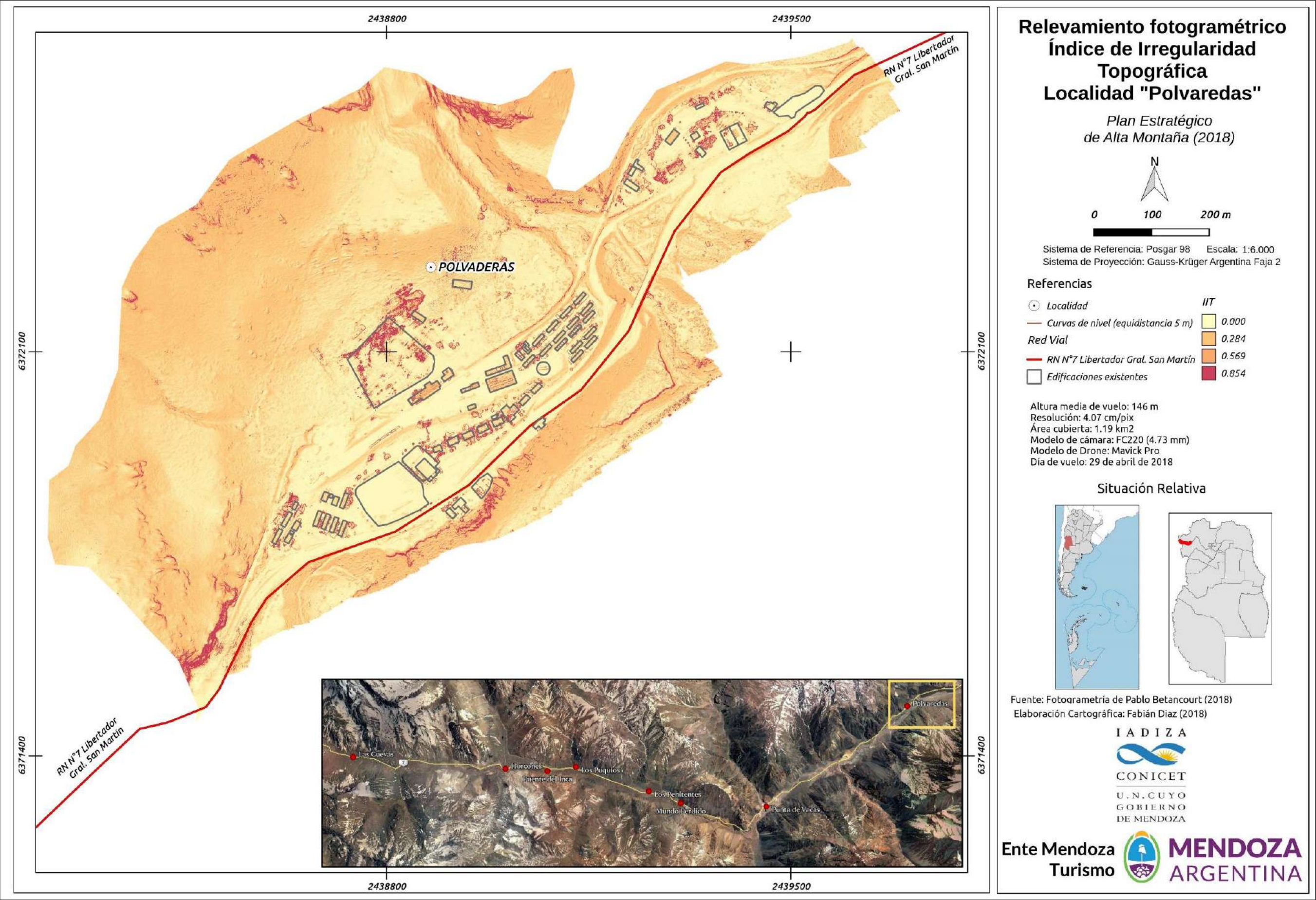
Figura 93. Relevamiento fotogramétrico. Índice de Irregularidad Topográfica. Localidad "Polvaredas".
