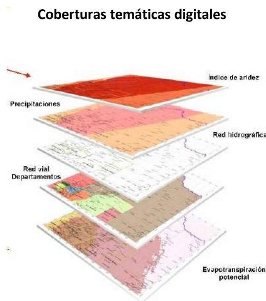
Figura 4. Esquema SIG de la Alta Montaña.
