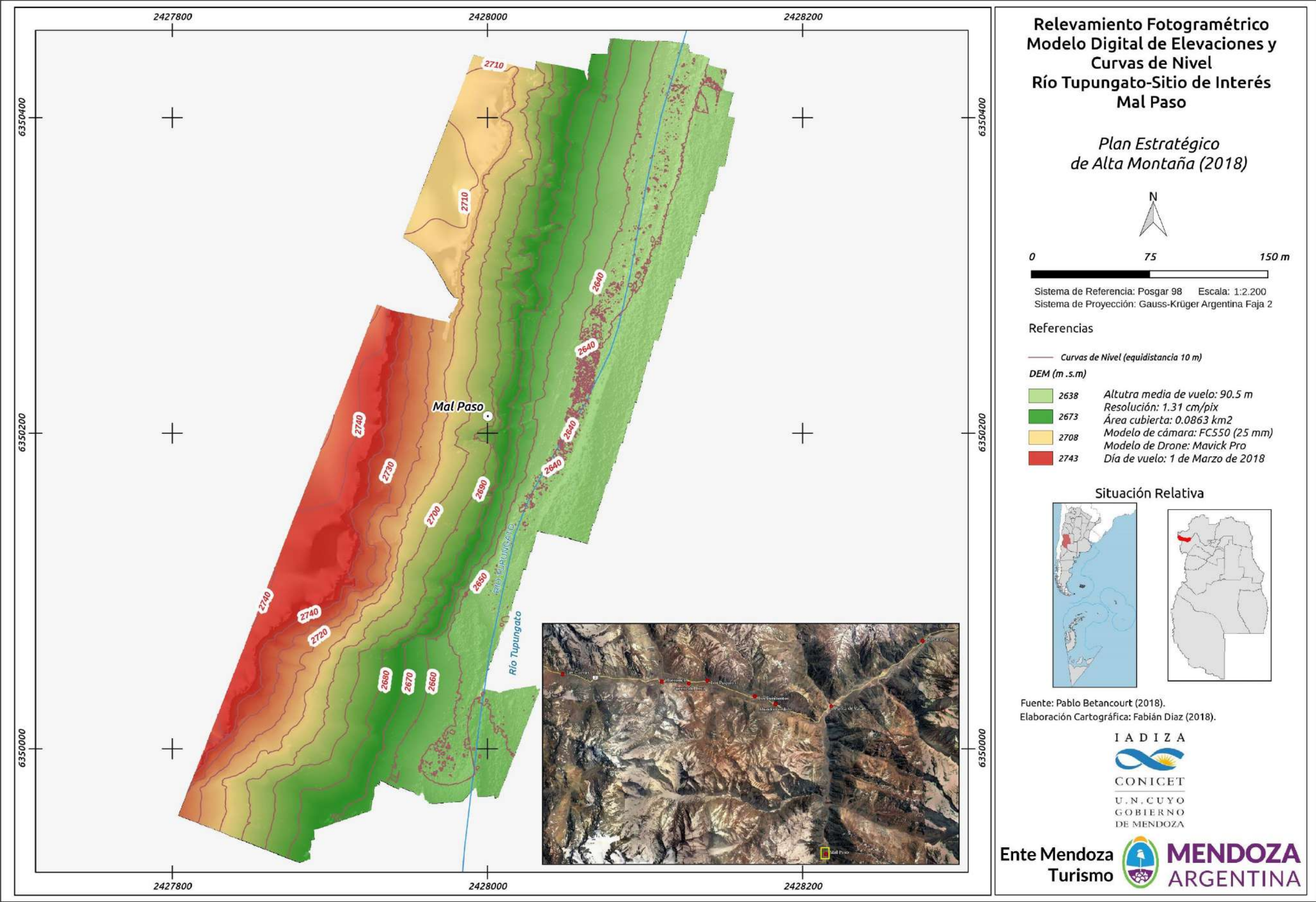
Figura 228. Relevamiento fotogramétrico. Modelo de Digital de Elevaciones (MDE) y Curvas de Nivel. Sitio natural de interés turístico “El mal paso”- Quebrada del río Tupungato.
