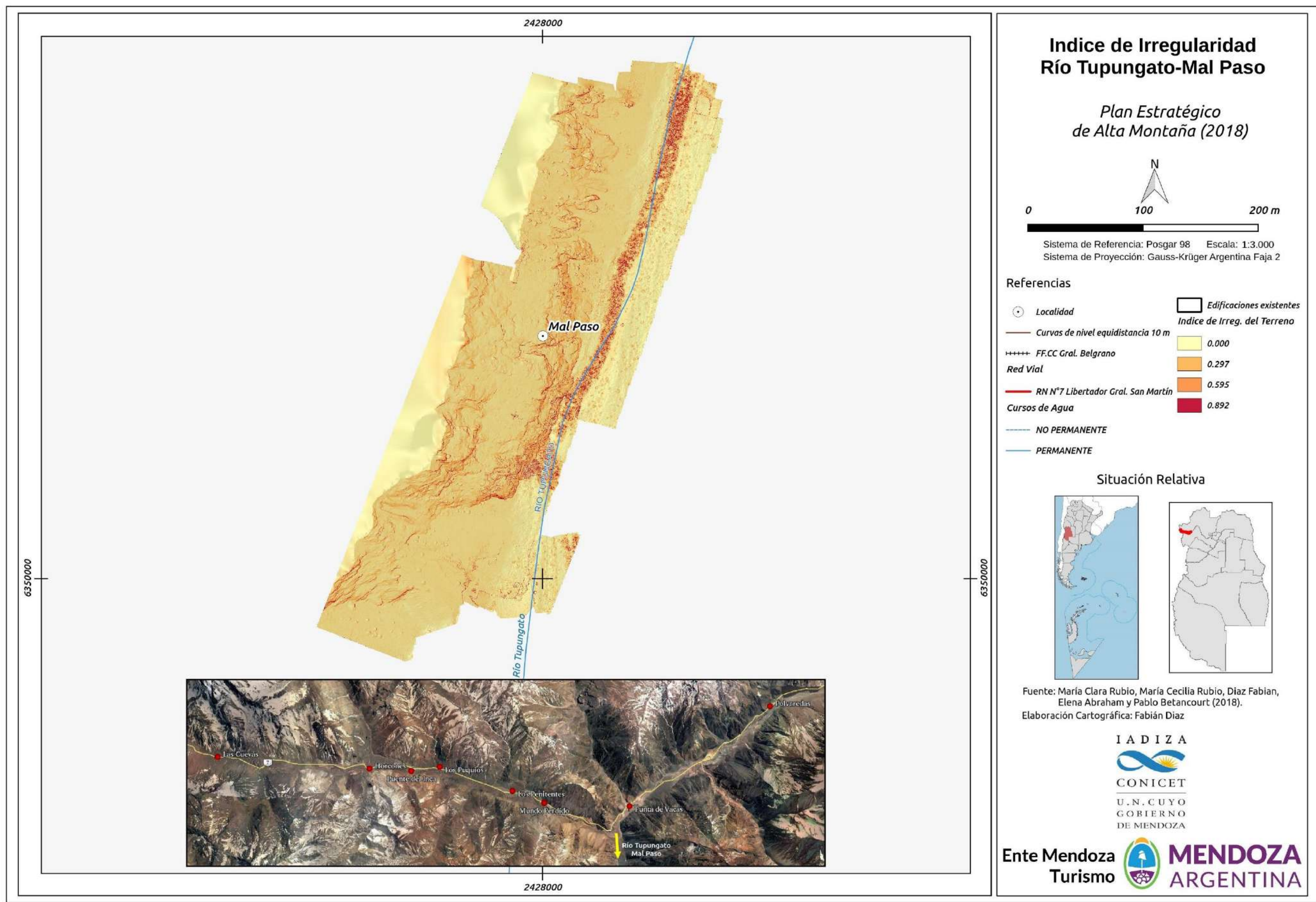
Figura 232. Relevamiento fotogramétrico. Índice de Irregularidad Topográfica. Sitio natural de interés turístico “El mal paso”- Quebrada del río Tupungato.
