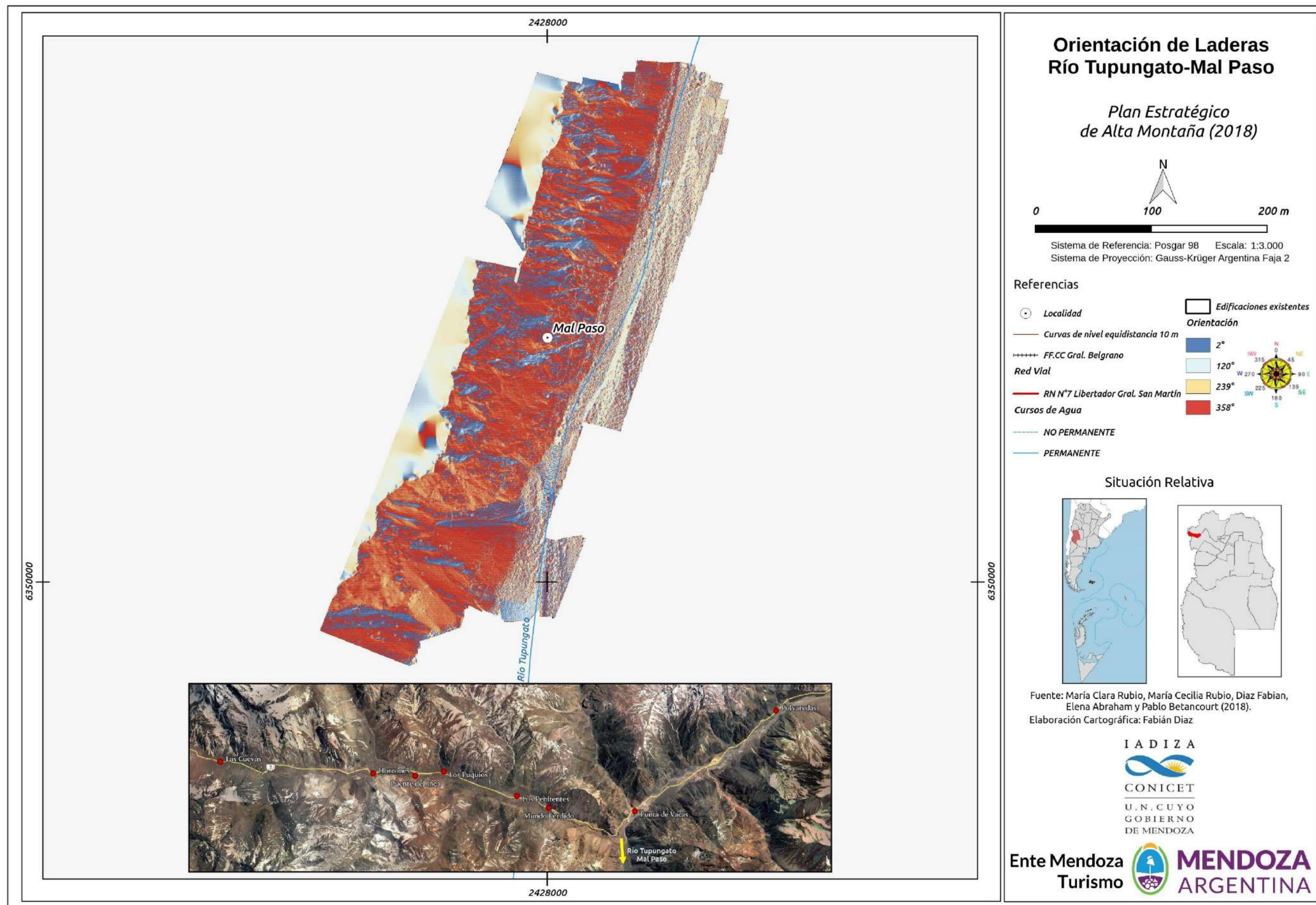
Figura 230. Relevamiento fotogramétrico. Orientación de laderas. Sitio natural de interés turístico “El mal paso”- Quebrada del río Tupungato.
