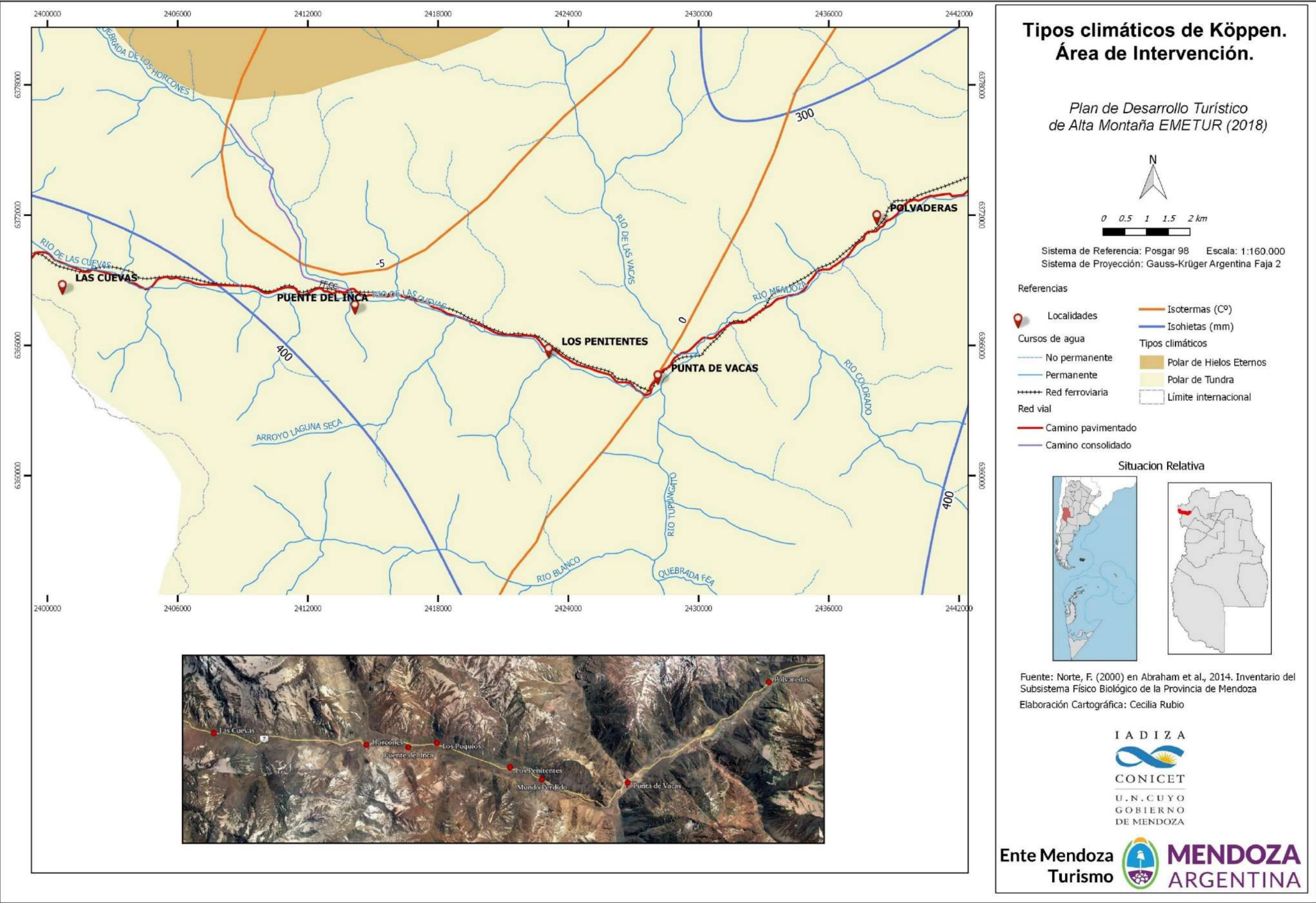
Figura 37. Tipos climáticos de Köppen del AI del PEAM. Fuente: Norte, F. (2000) en Abraham et al. (2014)
