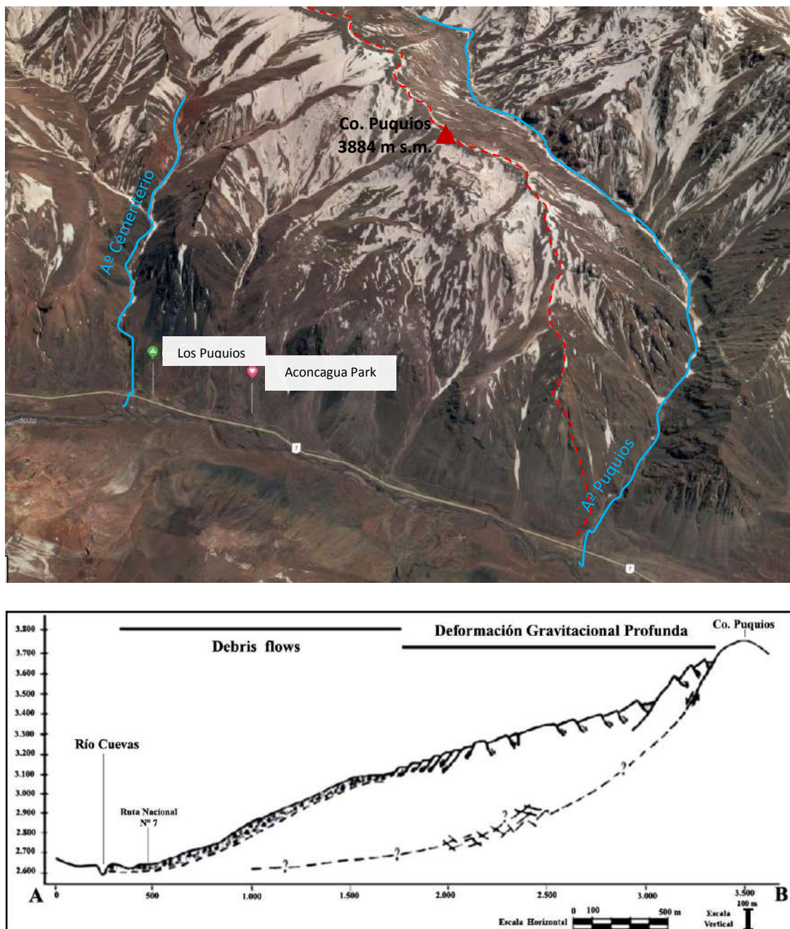
Figura 28. Imagen área de la zona de extensión del movimiento complejo y esquema del movimiento de deformación gravitacional profunda.
