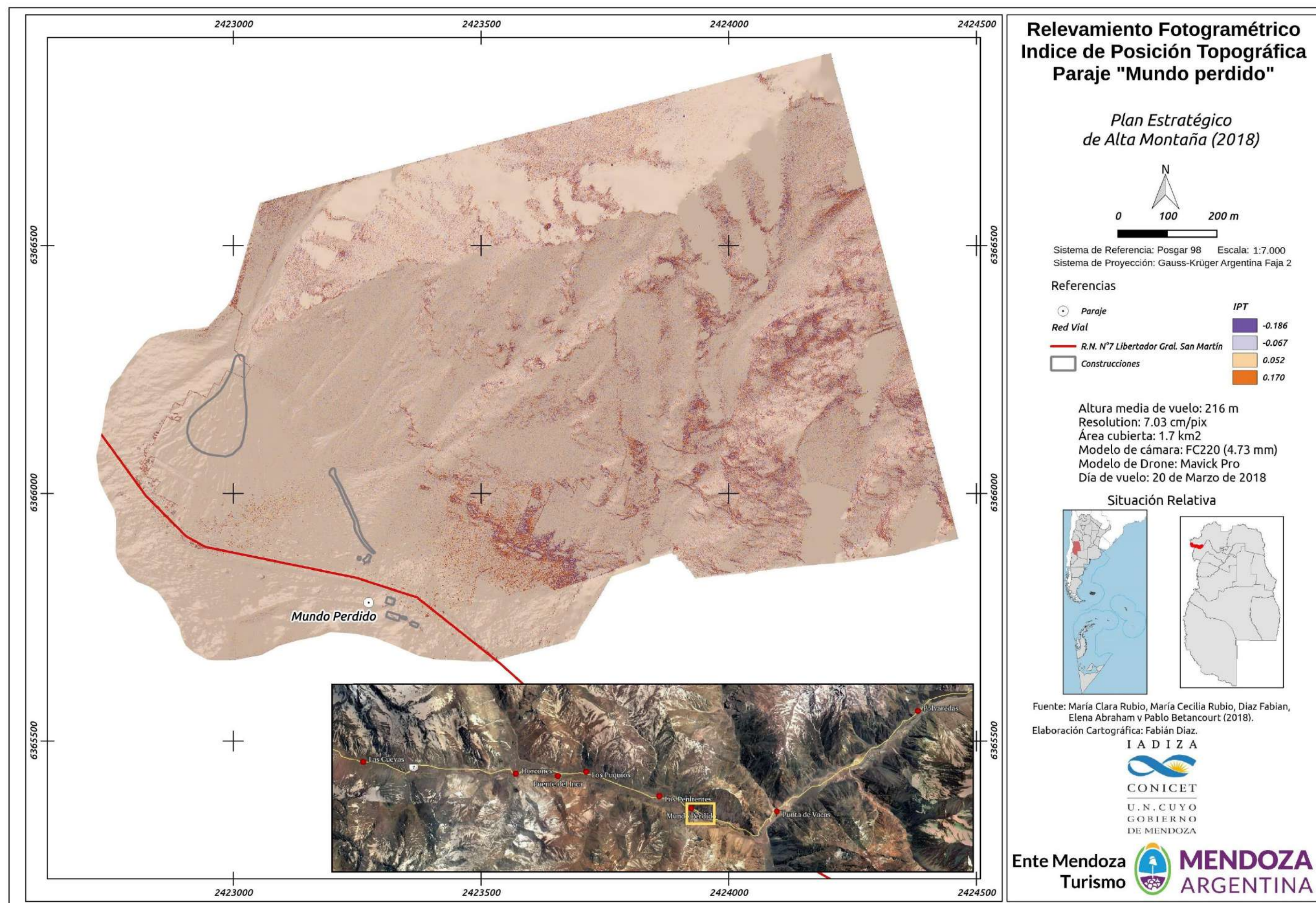
Figura 116. Relevamiento fotogramétrico. Índice de Posición Topográfica. Paraje Km 151 "Mundo perdido" y "Pircas".
