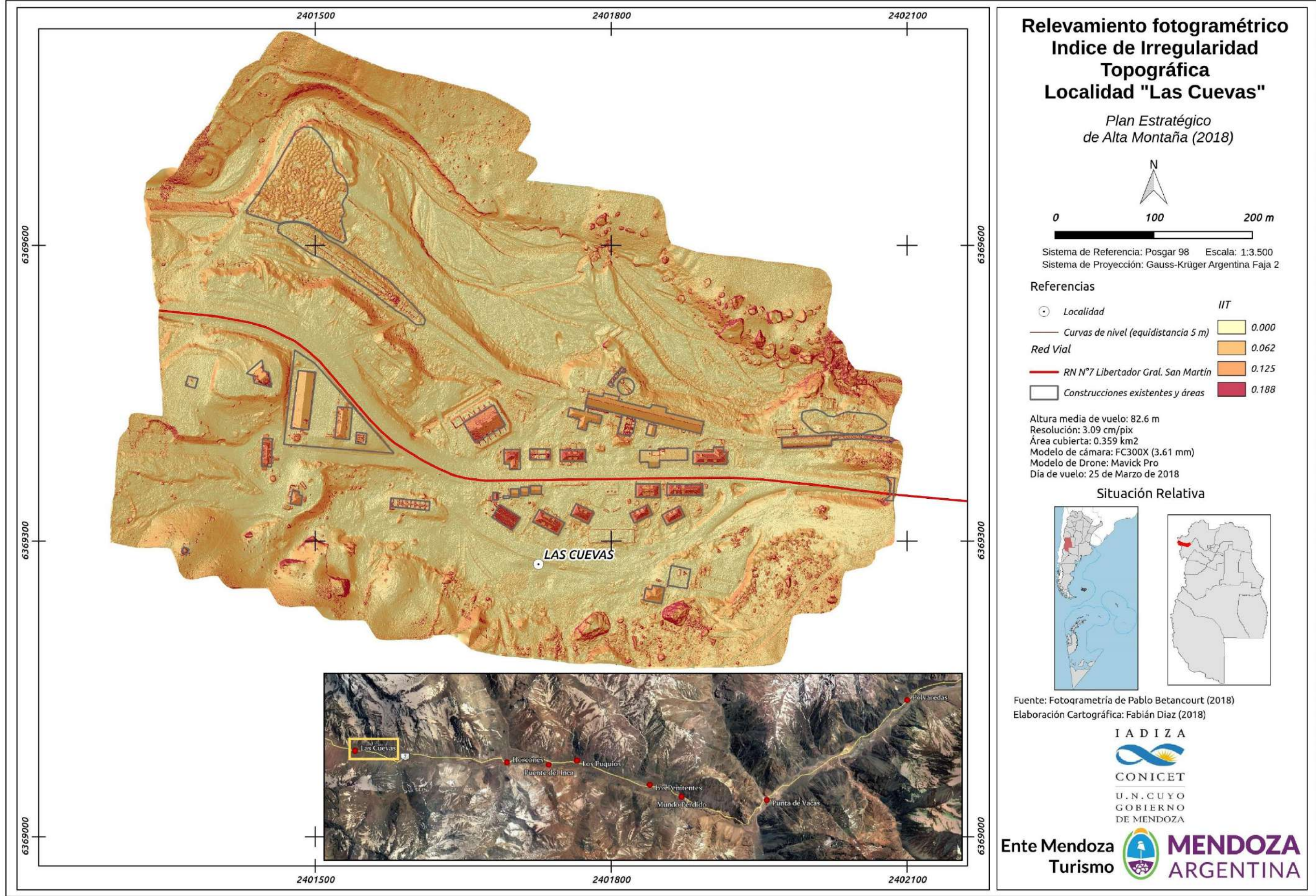
Figura 179. Relevamiento fotogramétrico. Índice de Irregularidad Topográfica. Localidad "Las Cuevas".
