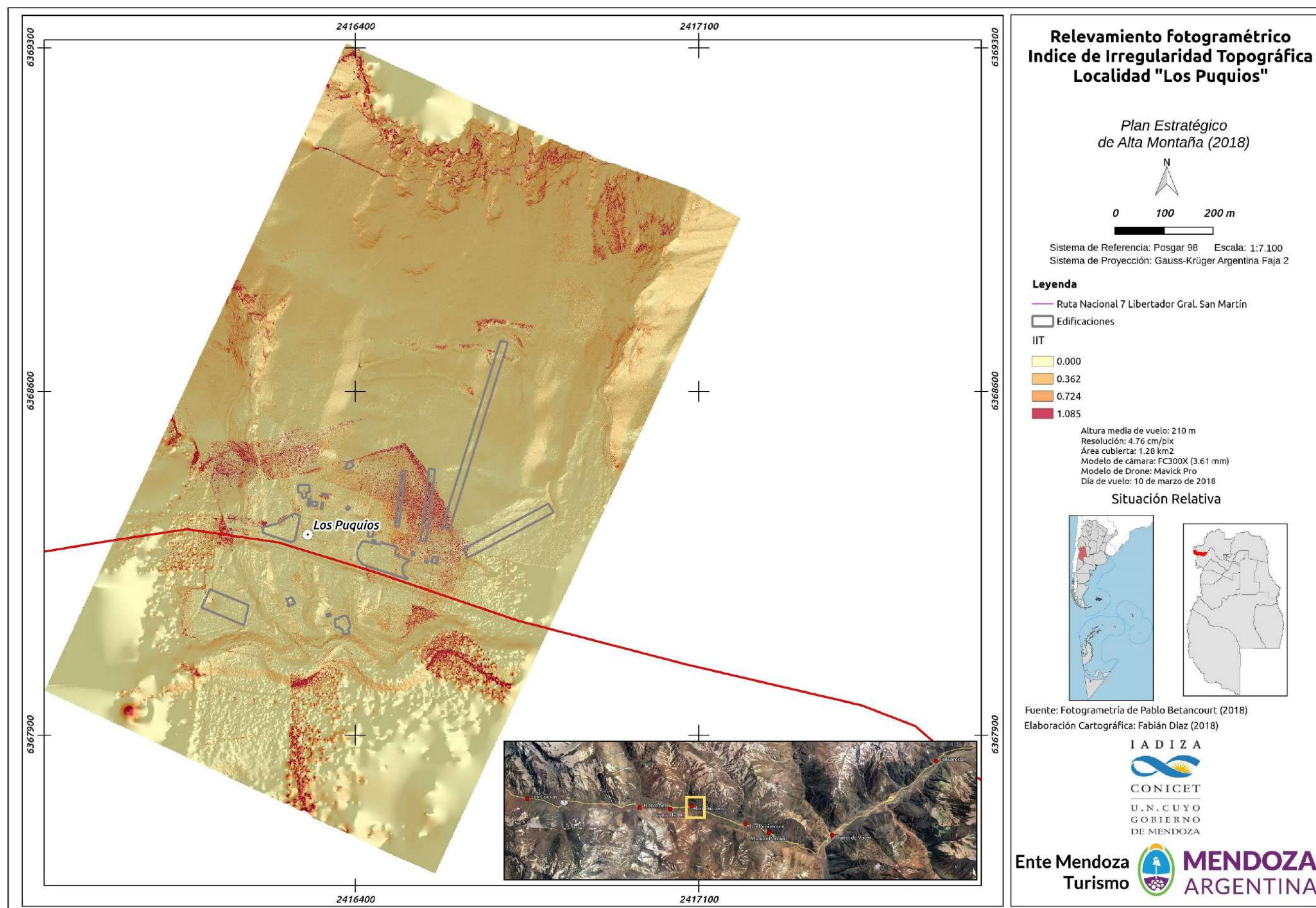
Figura 148. Relevamiento fotogramétrico. Índice de Irregularidad Topográfica. Paraje "Los Puquios".
