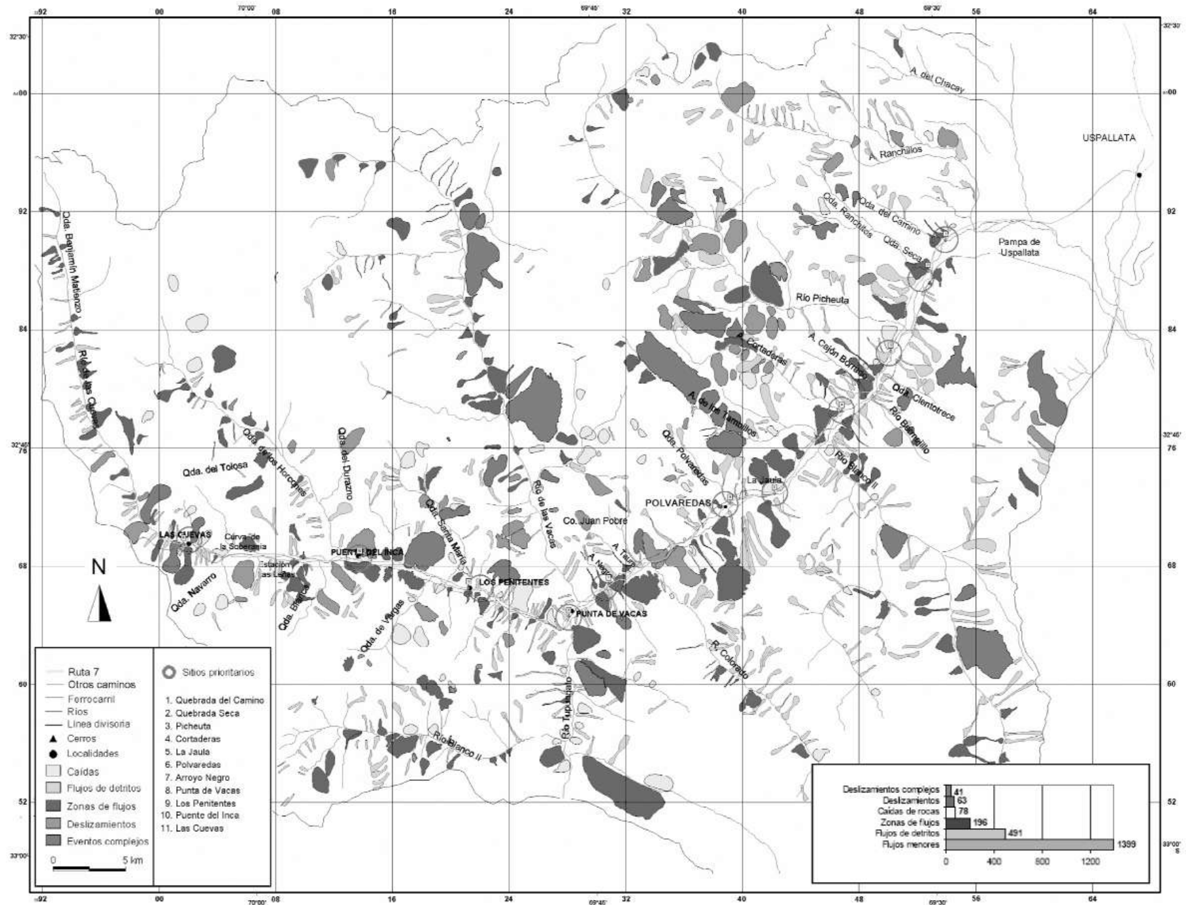
Figura 24. Mapa inventario de procesos de remoción en masa. Fuente: Moreiras (2009)
