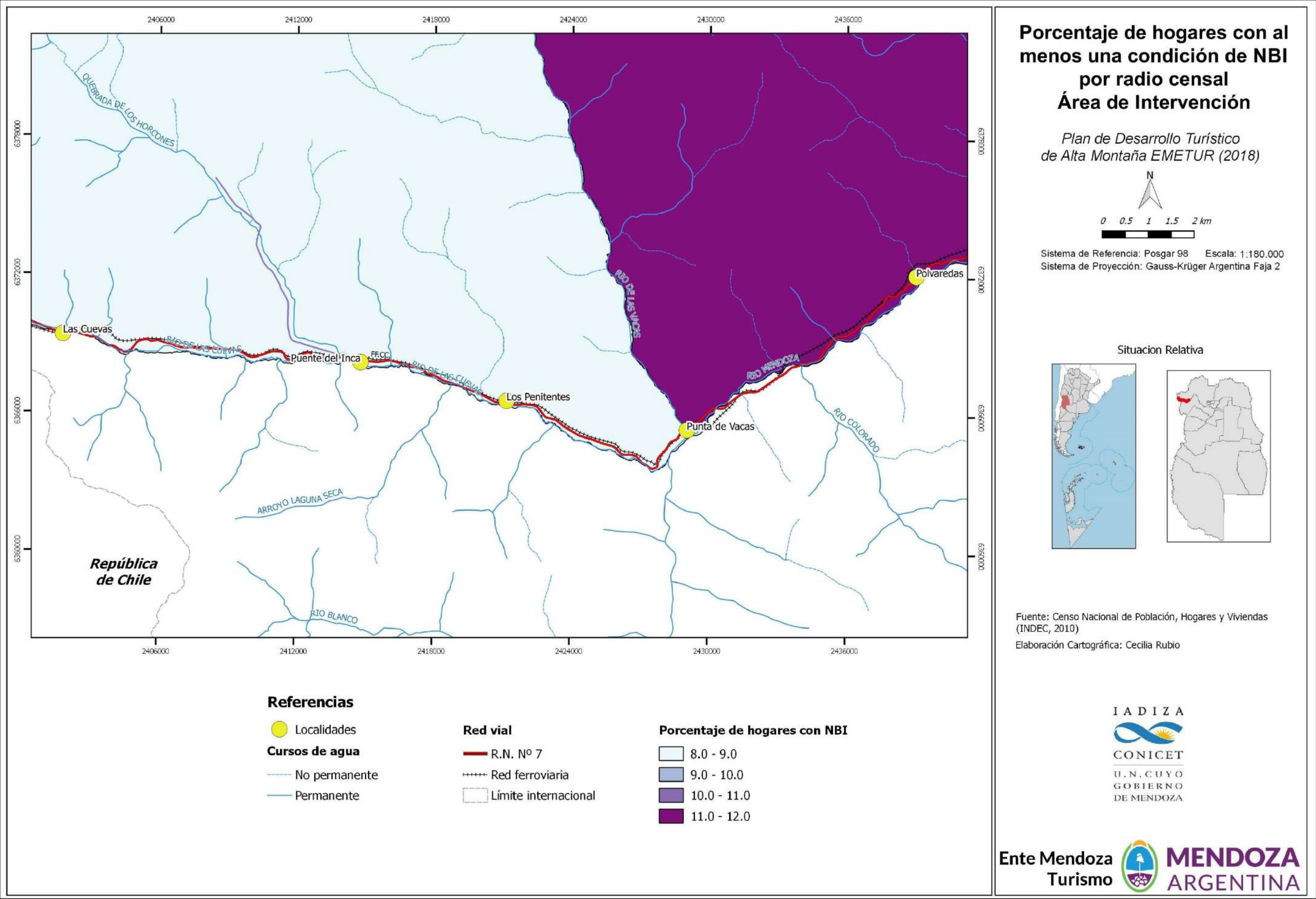
Figura 69. Porcentaje de hogares con al menos una condición de NBI por radio censal. Área de intervención del PEAM. Fuente: INDEC (2010)
