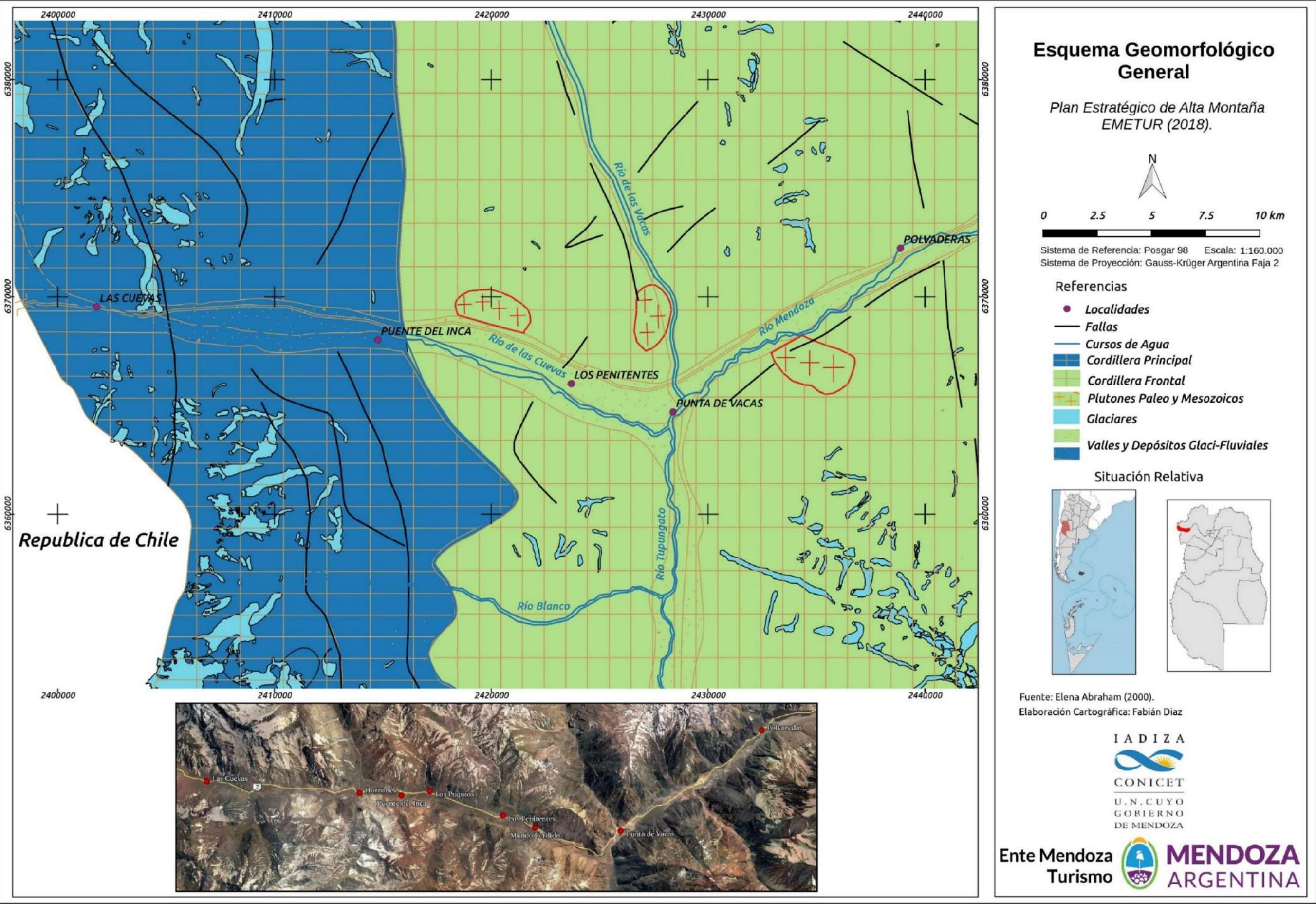
Figura 6. Esquema geomorfológico del AI del PEAM.
