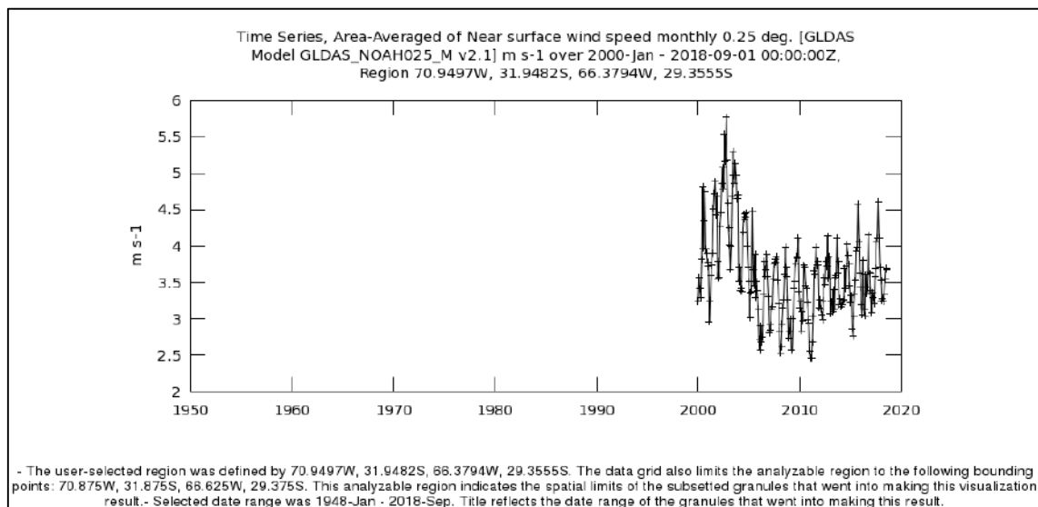
Figura 38. Velocidad de viento promedio mensual cercana a la superficie.
