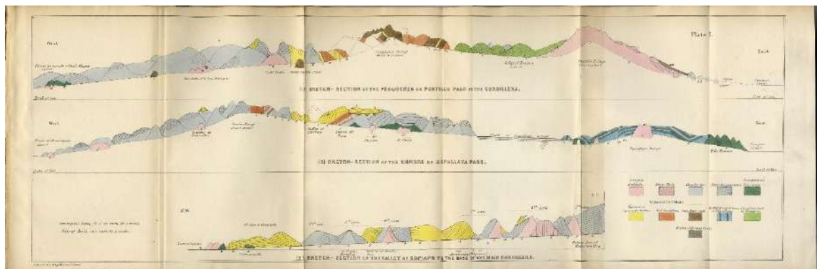
Figura 201. Secciones estructurales de la Cordillera de los Andes en los pasos de Piuquenes y de Uspallata
