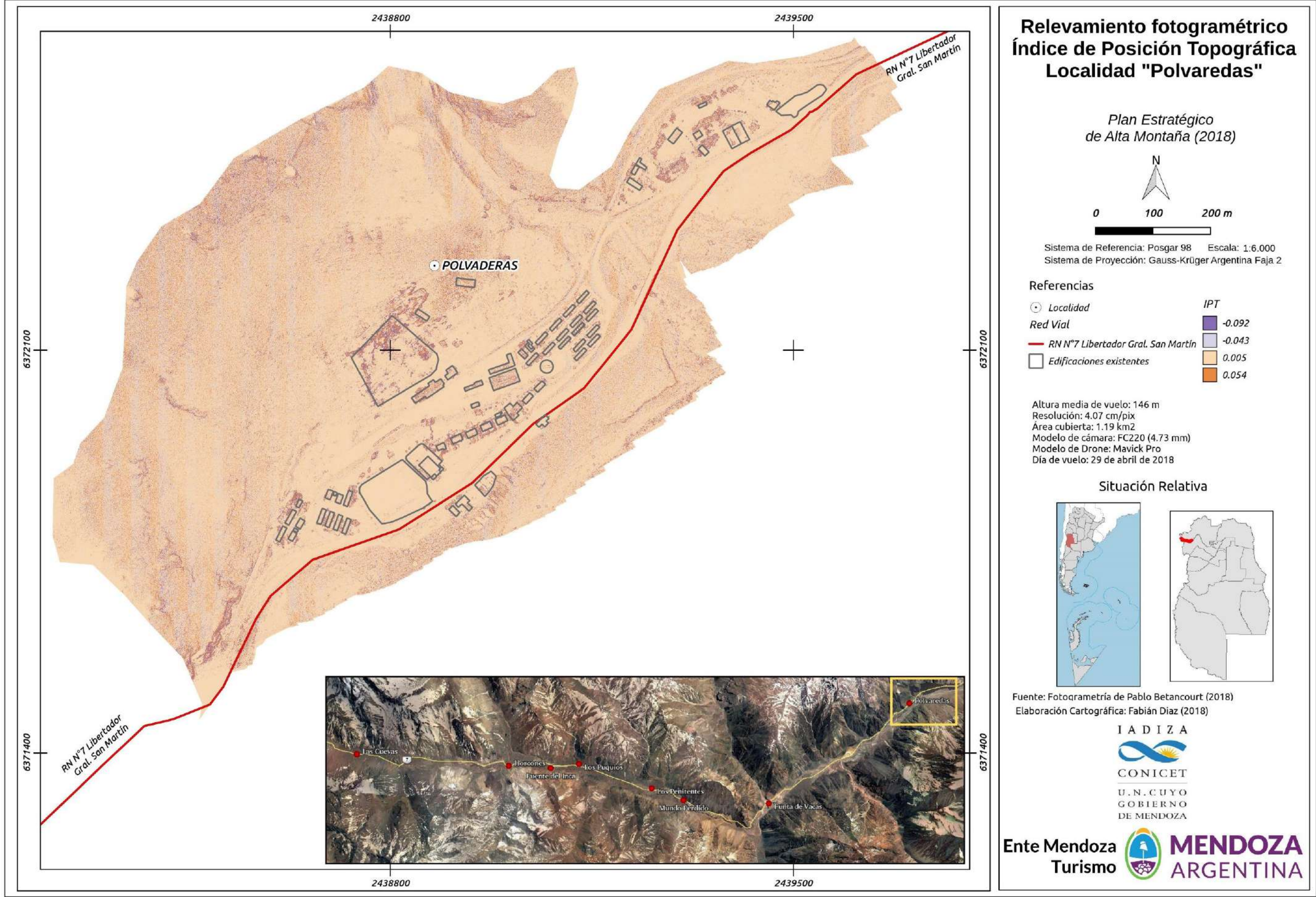
Figura 92. Relevamiento fotogramétrico. Índice de Posición Topográfica. Localidad "Polvaredas".
