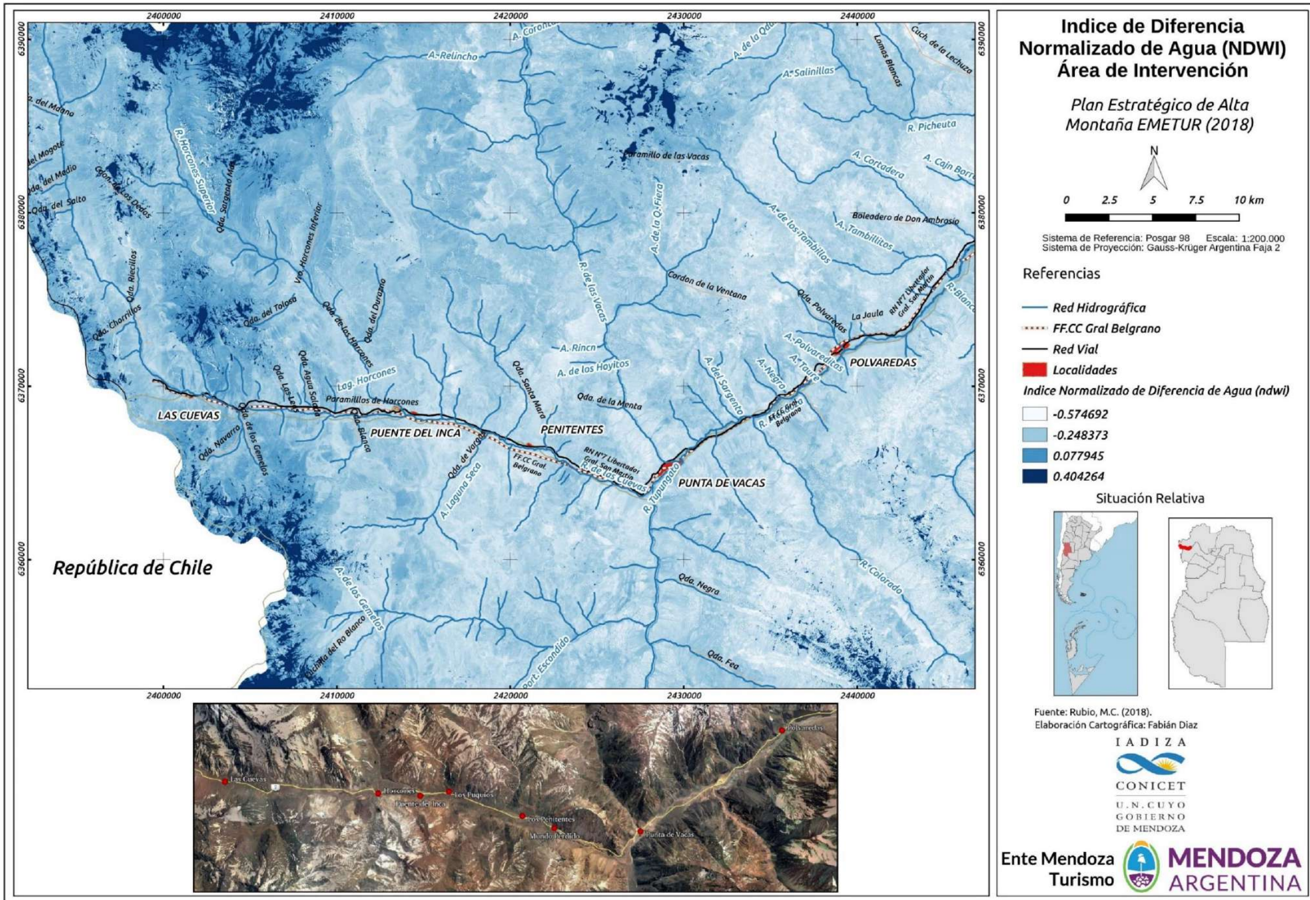
Figura 47. Aspectos hidrográficos del área de intervención del PEAM. Fuente: Rubio, M.C. (2018)
