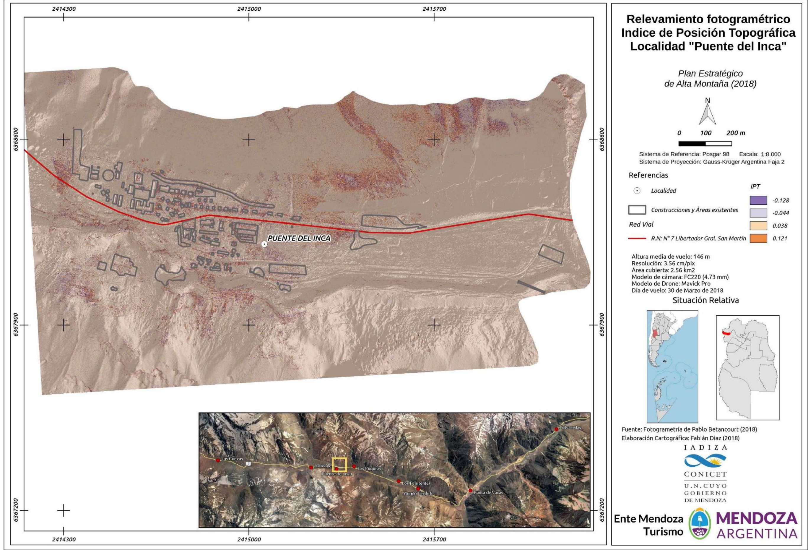
Figura 163. Relevamiento fotogramétrico. Índice de Posición Topográfica. Localidad "Puente del Inca".
