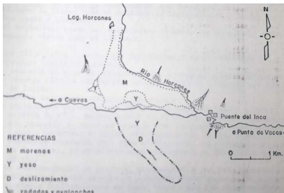
Figura 31. Principales accidentes por rodados, deslizamientos y avalanchas de nieve en la zona de la confluencia de los ríos de Los Horcones y de Las Cuevas.
